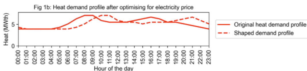
Figuur 4.7: Optimaliseren warmtevraag naar elektriciteitsprijs (Oxenaar & Butler, 2026).
