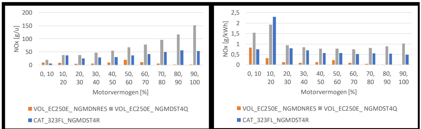
Figuur 5.1: Links: NO x -emissies in gram per uur als functie van de motorbelasting [%] voor de drie gemonitorde machines. Rechts: NO x -emissies in gram per kWh als functie van de motorbelasting [%] voor de drie gemonitorde machines.
