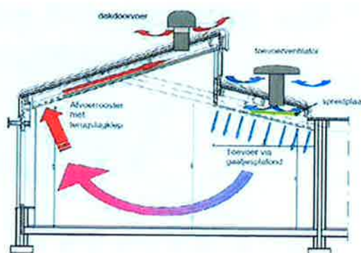
Systeemopzet voor klaslokaal met lessenaarsdak.
