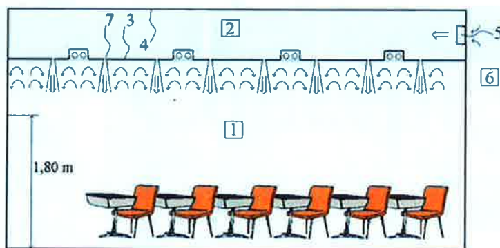
Principe van het plafond luchtdistributie concept.
