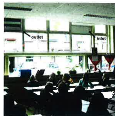
Frissescholen-concept met decentrale toe- en afvoer via de gevel.
