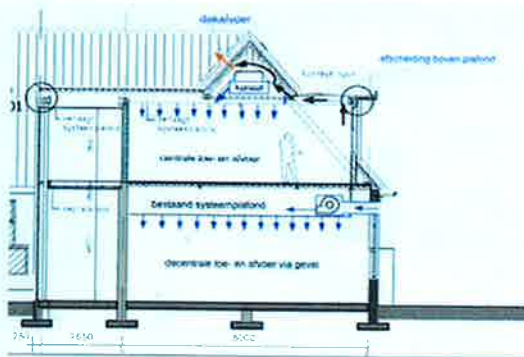
Frissescholen-concept met op 1 e etage centrale toe- en afvoer en op de begane grond decentrale toe- en afvoer via de gevel.
