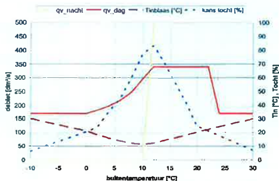
Benodigd debiet en tochtkans bij een klaslokaal met geveltoevoer.
