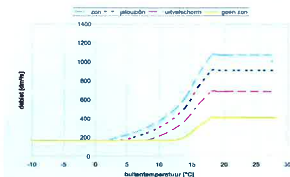
Effect van zoninstraling op vereiste ventilatiestroom per klaslokaal.
