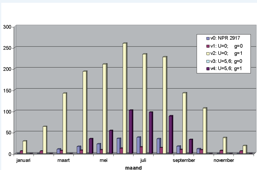
De koelbehoefte per maand in GJ voor de beschouwde varianten.
