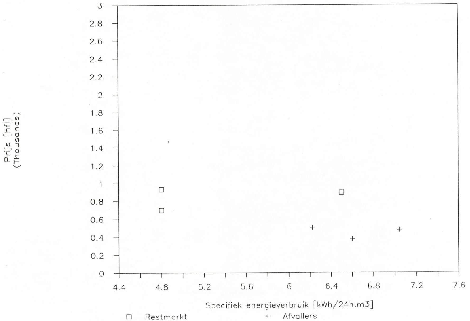
Figuur 21 Economisch gevolg van grenslijn 1 Vrijstaande koelkasten, 1*, volumecategorie 100 t/m 150 liter
