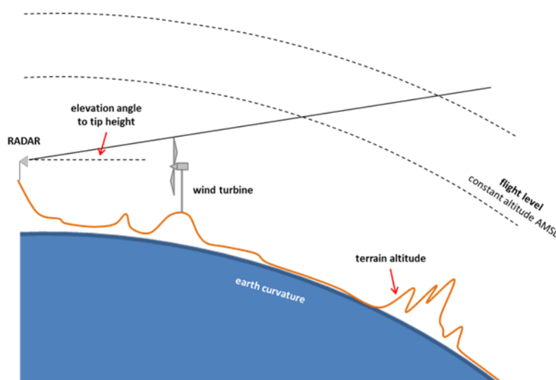
Figuur 21 Een overzicht van de algemene line-of-sight geometrie met een vaste azimuth. De elevatiehoek naar het hoogste punt van de turbine wordt aangegeven met een grijze lijn. Transponders signalen vanuit vliegtuigen boven deze lijn worden niet beïnvloed door de windturbine. Transponders van vliegtuigen onder deze lijn worden mogelijk beïnvloed door de turbine.
