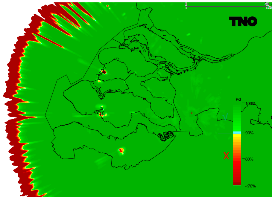
Figuur 35 De radardekking boven zuidwest Nederland op 1000 voet berekend met alleen de MASS radars en de TAR West.
