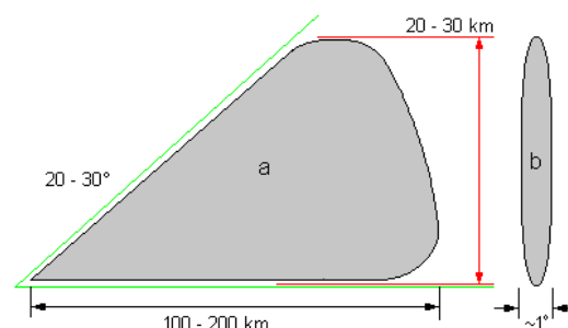
Figuur 2.1: Een vaanvormige bundel, de typische bundelvorm voor een rondzoekradar
