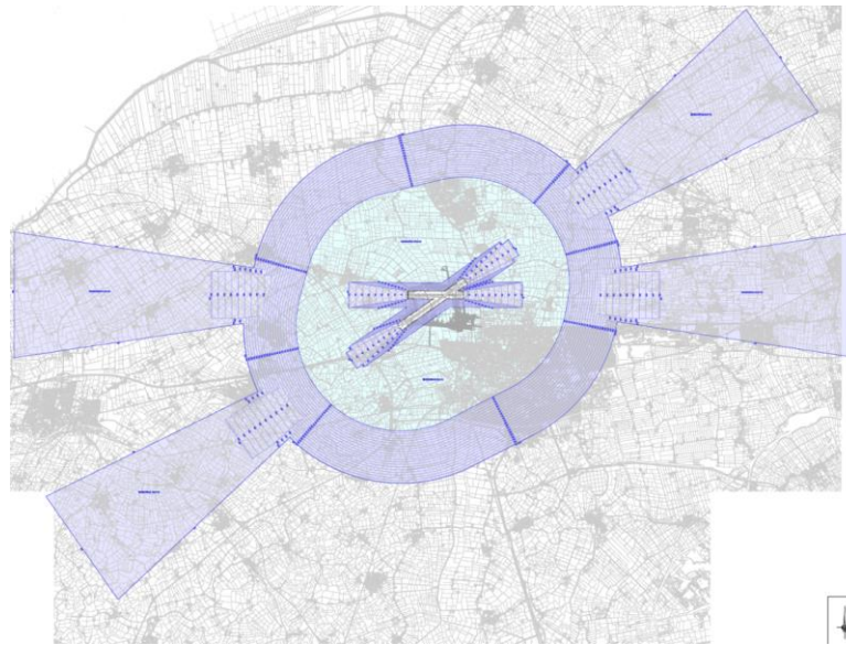
Figuur 31: Een voorbeeld van de ligging van de IHCS en funnels en de bouwhoogtebeperkingen daarbinnen voor in dit geval de vliegbasis Leeuwarden [Ministerie van Defensie].
