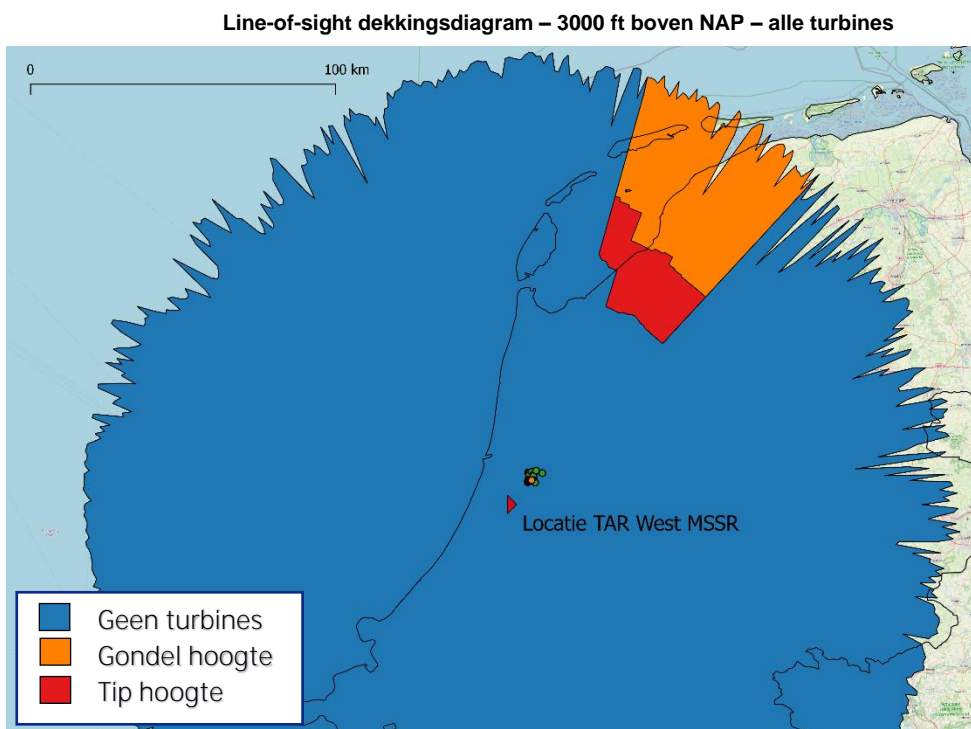
Figuur 47 Horizontaal line-of-sight dekkingdiagram op 3000 voet boven NAP gezien vanuit de secundaire radar. Zowel de bestaande windturbines als het bouwplan zijn in beschouwing genomen.
