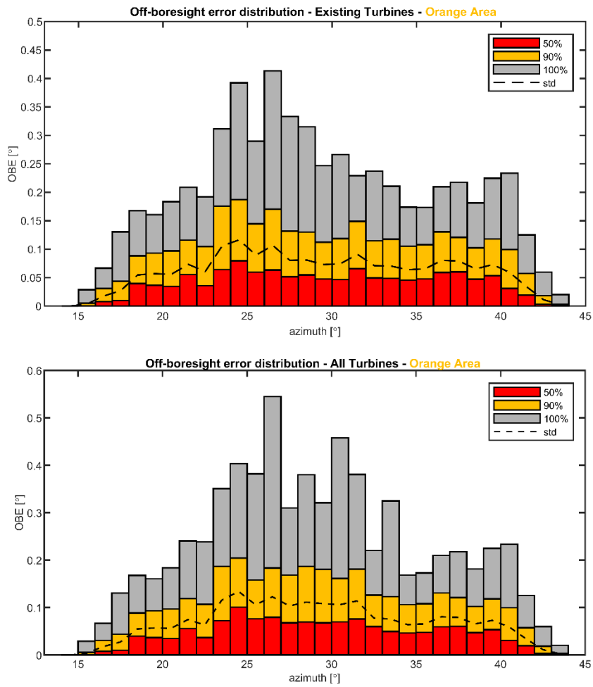
Figuur 33 Boven: de cumulatieve verdeling van de absolute peiling fout per azimuth sector van 1.0° wanneer alleen de bestaande turbines worden beschouwd. Voor elke azimuth sector worden de waarden van het 50 ste , 90 ste en 100 ste percentiel weergegeven, net als de standaard deviatie (1 \sigma ) van 68%, aangenomen dat de fout normaal verdeeld is. De maximale peilingshoek fout van de oranje zone van 0.41° komt voor bij een hoek van 26°-27°. In 90% van de gevallen is de peilingshoek fout in deze sector onder de 0.17° en in 50% van de gevallen onder de 0.06°. Onder: Hetzelfde als de bovenste figuur, maar nu voor zowel de bestaande turbines als het bouwplan. De maximale absolute fout van 0.54° komt voor in de azimuth sector van 26°-27°. Het 90 ste percentiel is 0.18° en het 50 ste percentiel is 0.08°.
