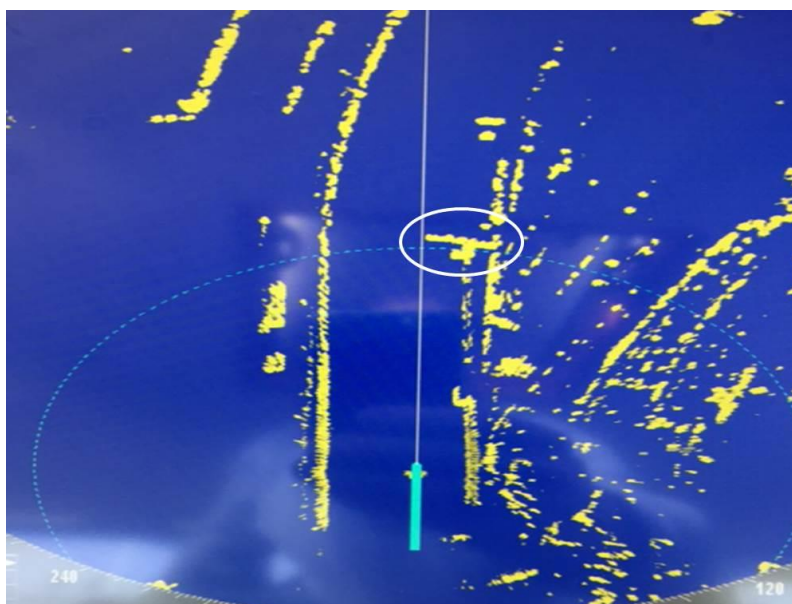
Figuur 68: Verbreiding windturbine in de praktijk langs het Hartelkanaal. De windturbine is zichtbaar in de witte cirkel. De windturbine staat op de waterlijn, dus de wieken reiken in dit voorbeeld ook zonder verbreiding al over de vaarweg.
