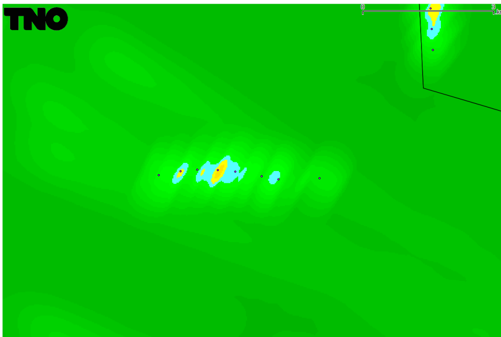
Figuur 40 De berekende detectiekans van de ASR-M radar bij Kleine Brogel boven een windpark op een doelhoogte van 1000 voet waarbij de VCC techniek wel is geactiveerd.
