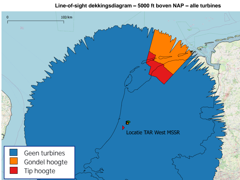
Figuur 49 Horizontaal line-of-sight dekking diagram voor een doelwit op 5000 voet boven NAP gezien vanuit de secundaire radar. Zowel de bestaande windturbines als het bouwplan zijn in beschouwing genomen.
