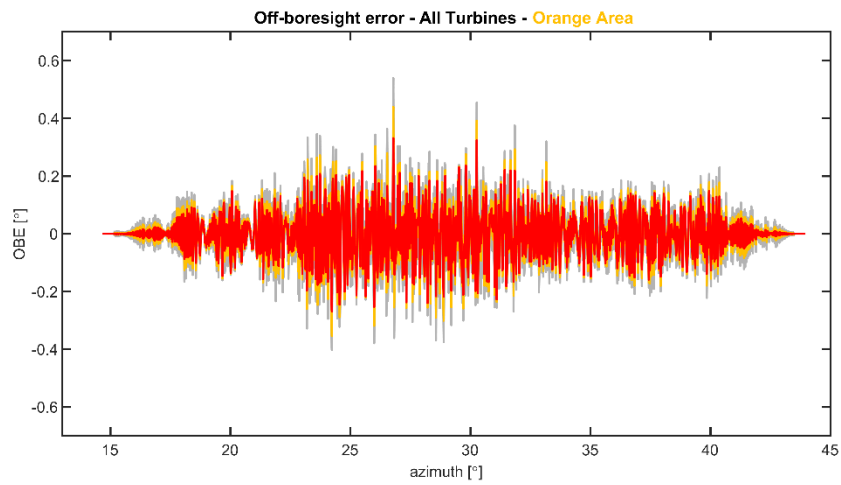
Figuur 32 Boven: de peilingshoek fout als functie van azimuth voor de bestaande turbines voor de secundaire radar, in de oranje zone. De maximale absolute fout voor de oranje zones is 0.41^\circ . Onder: hetzelfde als boven, maar nu voor zowel de bestaande turbines als het bouwplan. De maximale absolute fout is hier 0.54^\circ .
