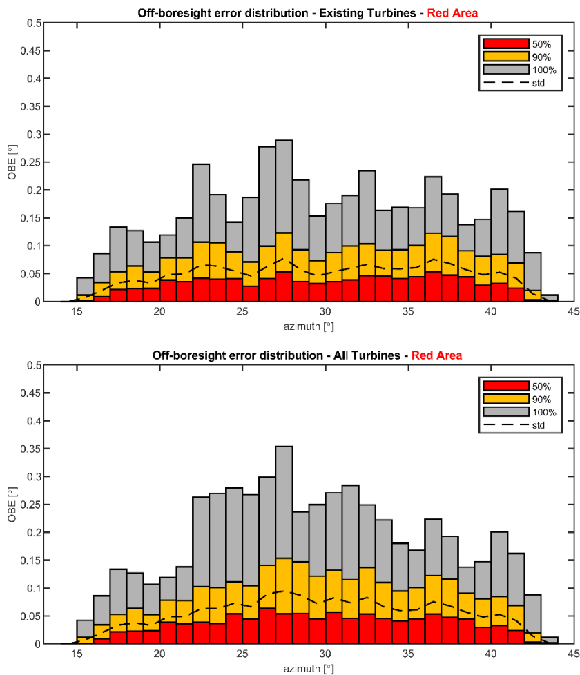
Figuur 35 Boven: de cumulatieve verdeling van de absolute peiling fout per azimuth sector van 1.0° wanneer alleen de bestaande turbines worden beschouwd. Voor elke azimuth sector worden de waarden van het 50 ste , 90 ste en 100 ste percentiel weergegeven, net als de standaard deviatie (1 \sigma ) van 68%, aangenomen dat de fout normaal verdeeld is. De maximale peilingshoek fout van de rode zone van 0.29° komt voor bij een hoek van 27°-28°. In 90% van de gevallen is de peilingshoek fout in deze sector onder de 0.12° en in 50% van de gevallen onder de 0.05°. Onder: Hetzelfde als de bovenste figuur, maar nu voor zowel de bestaande turbines als het bouwplan. De maximale absolute fout van 0.35° komt voor in de azimuth sector van 27°-28°. Het 90 ste percentiel is 0.15° en het 50 ste percentiel is 0.05°
