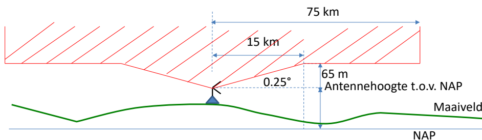
Figuur 9: Het hoogteprofiel (niet op schaal) voor windturbines. Als de tip van de wijk door het profiel steekt dient een toetsing plaats te vinden.
