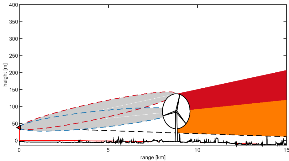
Figuur 23 Line-of-sight van de secundaire radar naar de dichtstbijzijnde geplande windturbine. De windturbine staat volledig in het zicht van de radar.
