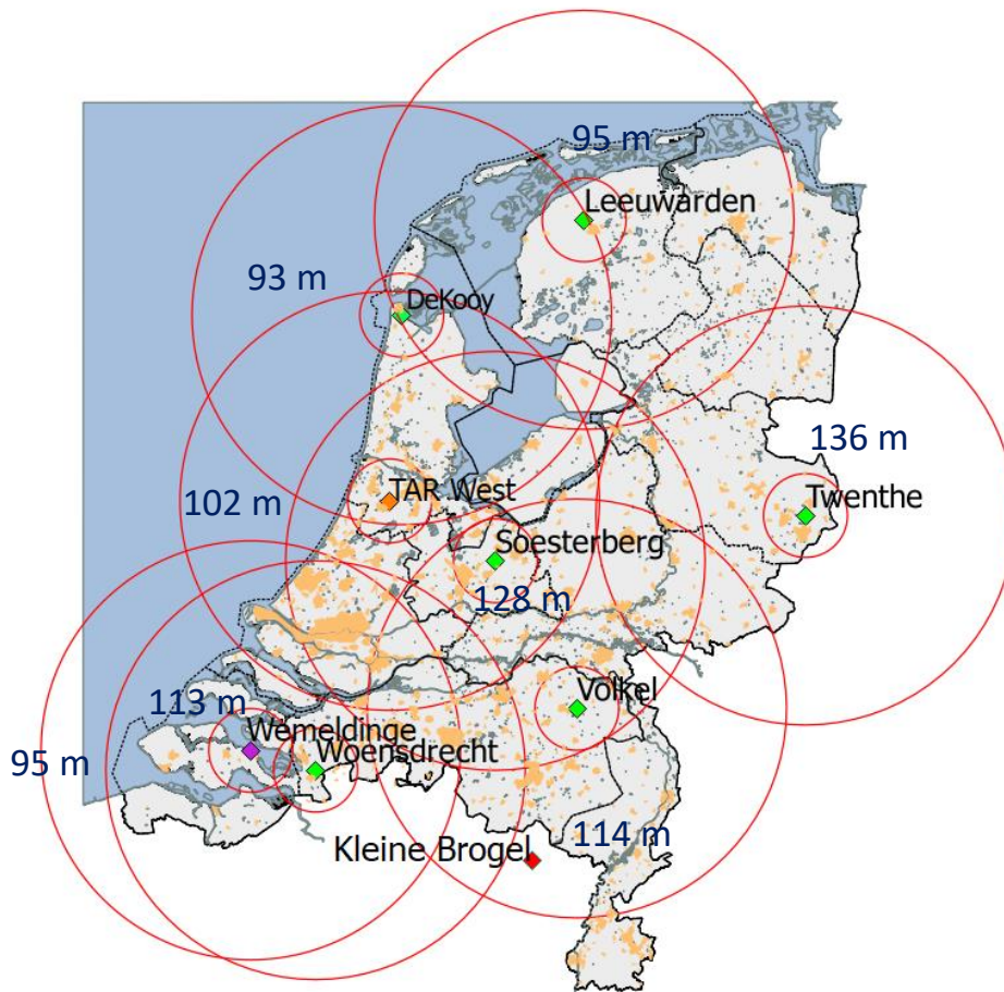
Figuur 10: De locaties van de zes MASS verkeersleidingsradars (groene ruit), de TAR West bij Schiphol (oranje ruit) en de Scantier 4002 infill radar bij Wemeldinge (paarse ruit) met daaromheen de 15 en 75 km cirkels. De getallen in de cirkels geven de tiphoogtes weer waarboven de toetsingsplicht geldt. In het overlapegebieden geldt de laagste tiphoogte.
