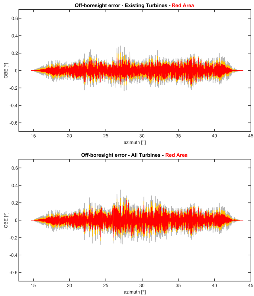
Figuur 34 Boven: de peilingsfout als functie van azimut voor de bestaande turbines voor de secundaire radar, in de rode zone. De maximale absolute fout voor de rode zones is 0.28°. Onder: hetzelfde als boven, maar nu voor zowel de bestaande turbines als het bouwplan. De maximale absolute fout is hier 0.35°.
