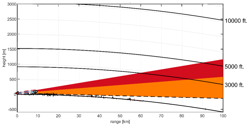
Figuur 24 Line-of-sight van secundaire radar, maar nu doorgetrokken tot 100 km vanaf de radar. De rode lijn geeft een indicatie op welke vlieghoogte de verstoring van het windpark nog van invloed is. Op 100 km van de radar zal de peiling van vliegtuigen tot een hoogte van circa 1750 m beïnvloed worden. Zonder de turbine zou dit een hoogte zijn van circa 450 m.
