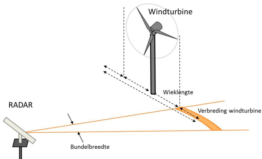
Figuur 67: Illustratie van doelverbreiding vanwege reflecties op de wijk van een windturbine.
