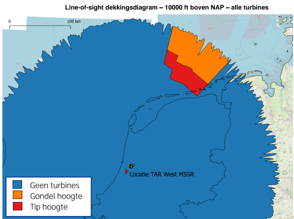
Figuur 51 Horizontaal line-of-sight dekking diagram voor een doelwit op 10000 voet boven NAP gezien vanuit de secundaire radar. Zowel de bestaande windturbines als het bouwplan zijn in beschouwing genomen.
