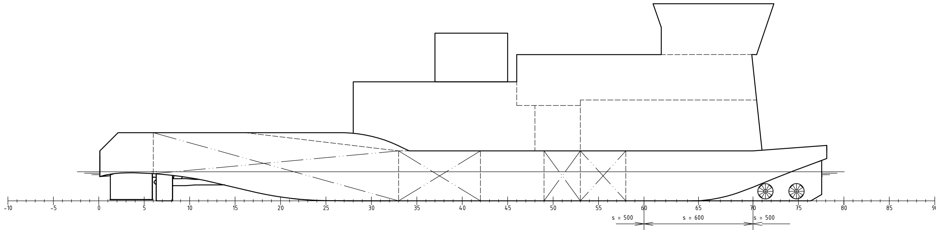
5.50 [m] BB
