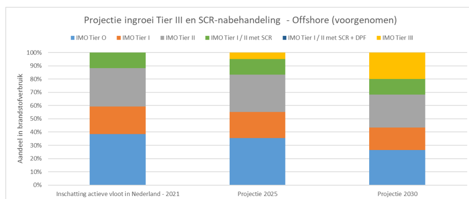
Figuur 15: Projectie van ingroei Tier III en SCR-nabehandeling bij schepen voor de aanleg van op zee en andere wind op zee activiteiten.
