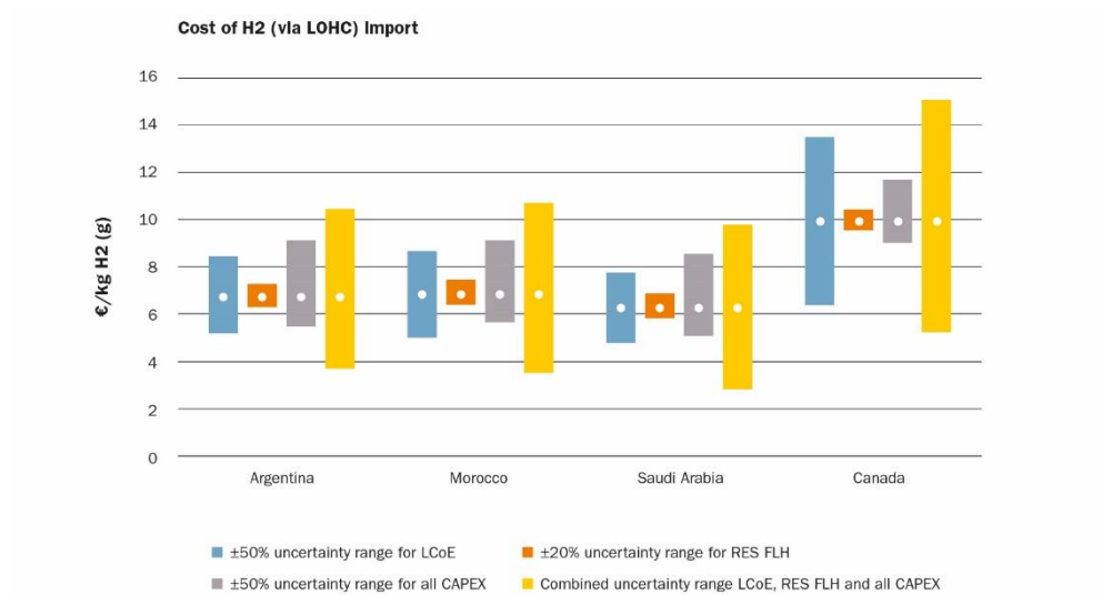
Figuur 13 Import van waterstof via LOHC
