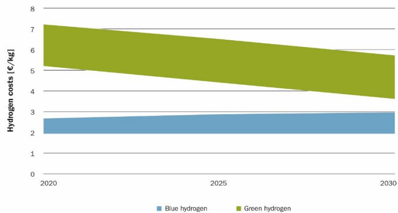
Figuur 6 Vergelijking van productiekosten van groene en blauwe waterstof in Nederland.
