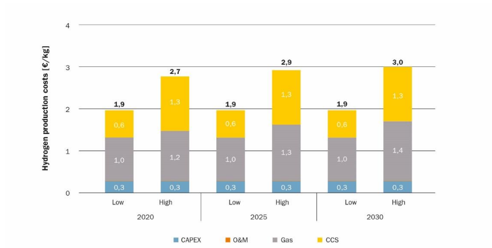
Figuur 5 Productiekosten van blauwe waterstof in Nederland.
