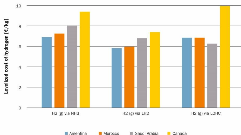
Figuur 10 Kosten van waterstof vanuit diverse landen en op diverse manieren geïmporteerd en in Nederland omgezet naar gasvormig waterstof op 70 bar.
