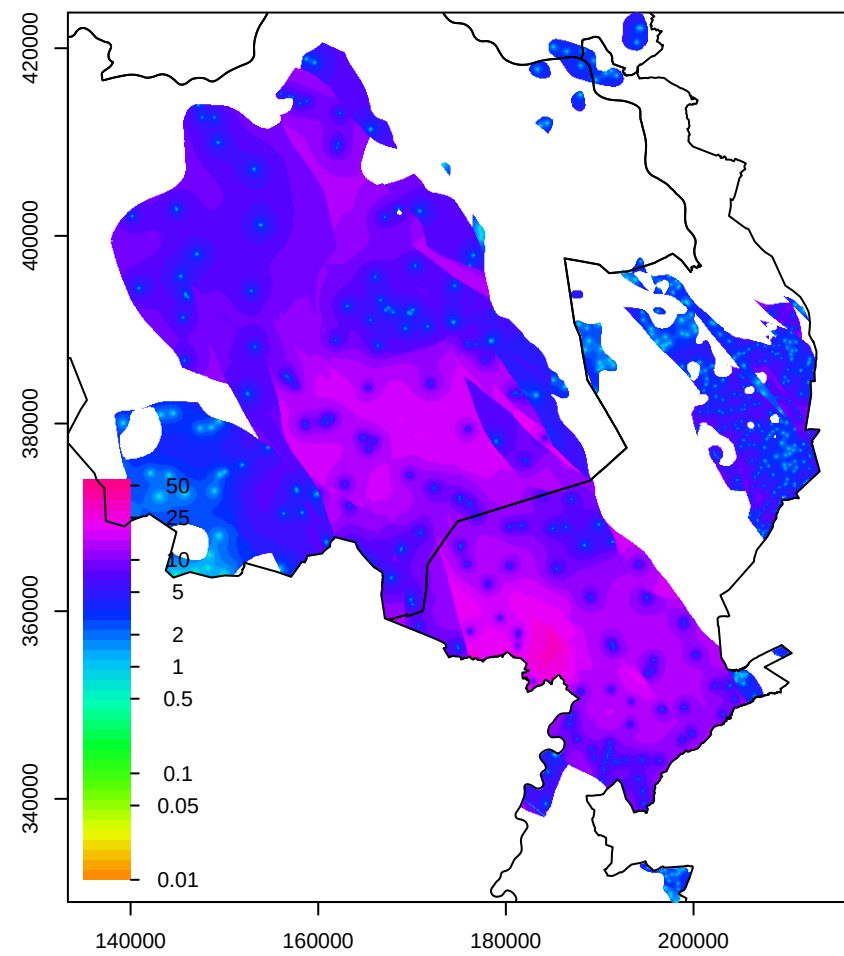
Kik1 std dikte
