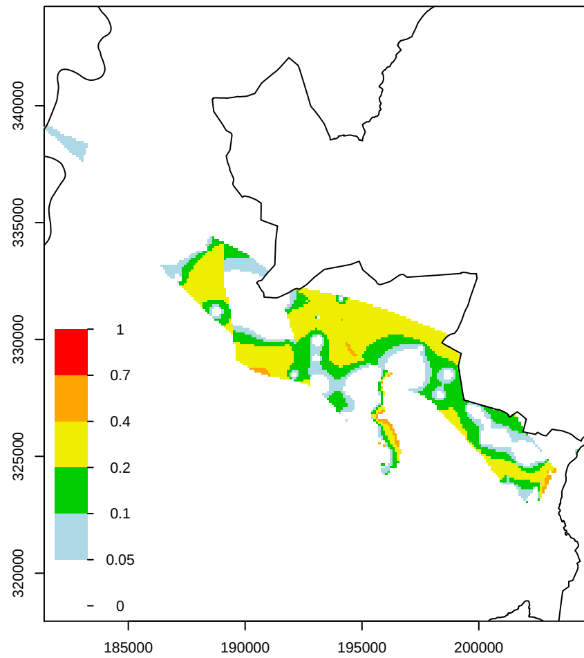
Vib1 kans op negatieve dikte
