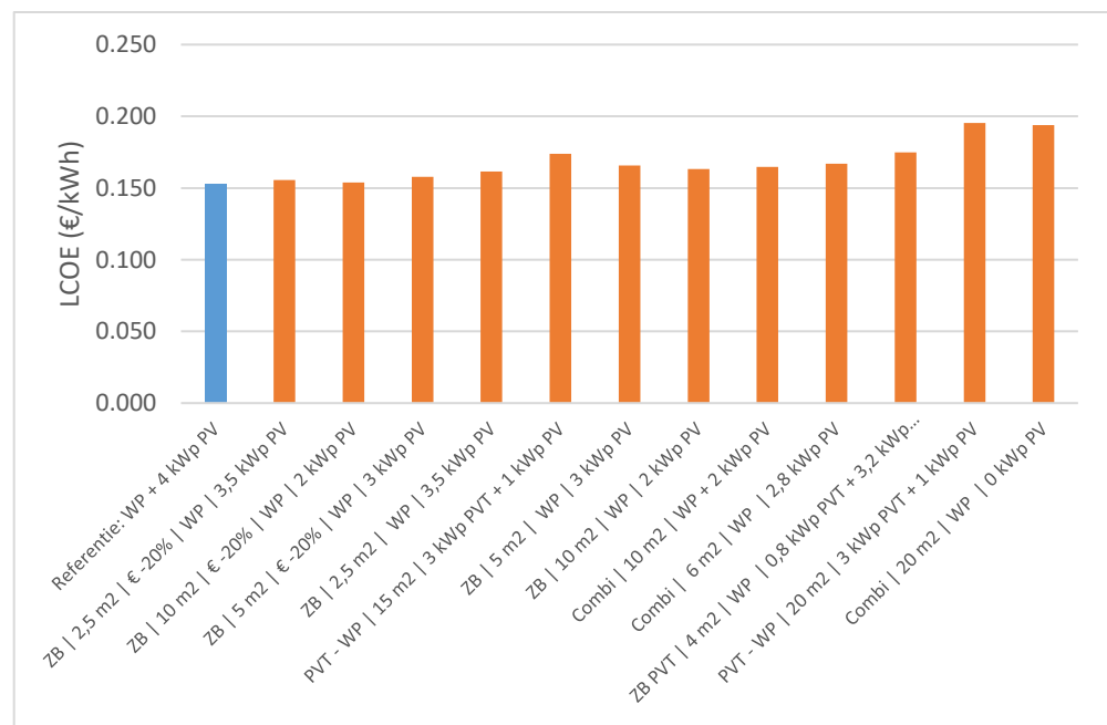
Figuur 4.6 LCOE voor warmtepomp - zonnepanelen
