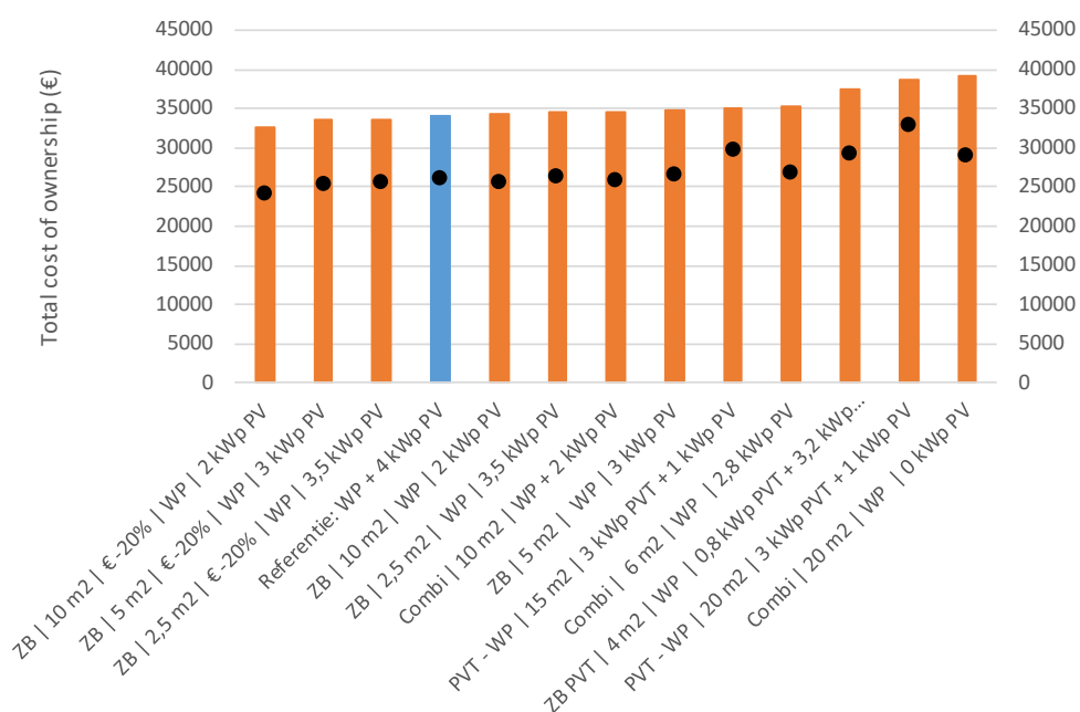
Figuur 4.7 Total cost of ownership voor referentiesysteem (warmtepomp met 4 kWp PV) en zonnewarmtesystemen met naverwarming door een warmtepomp. ZB = zonneboiler (alleen tapwater), Combi = combisysteem, PVT – WP = PVT-systeem als bron voor de warmtepomp
