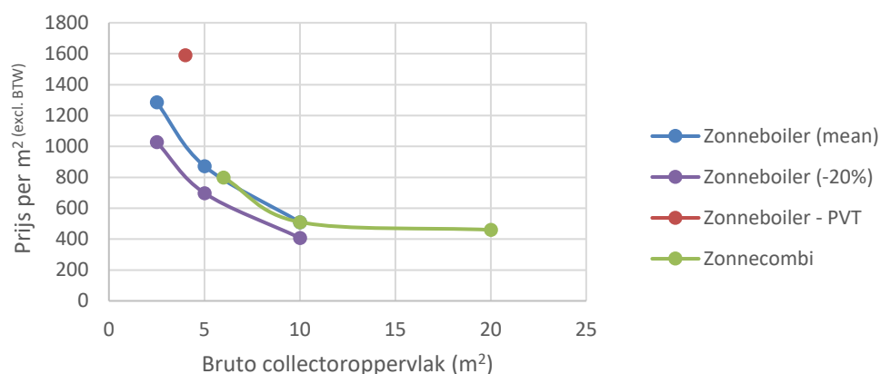
Figuur 3.6 Prijs per m² bruto collectoroppervlak voor verschillende systemen (excl. btw)
