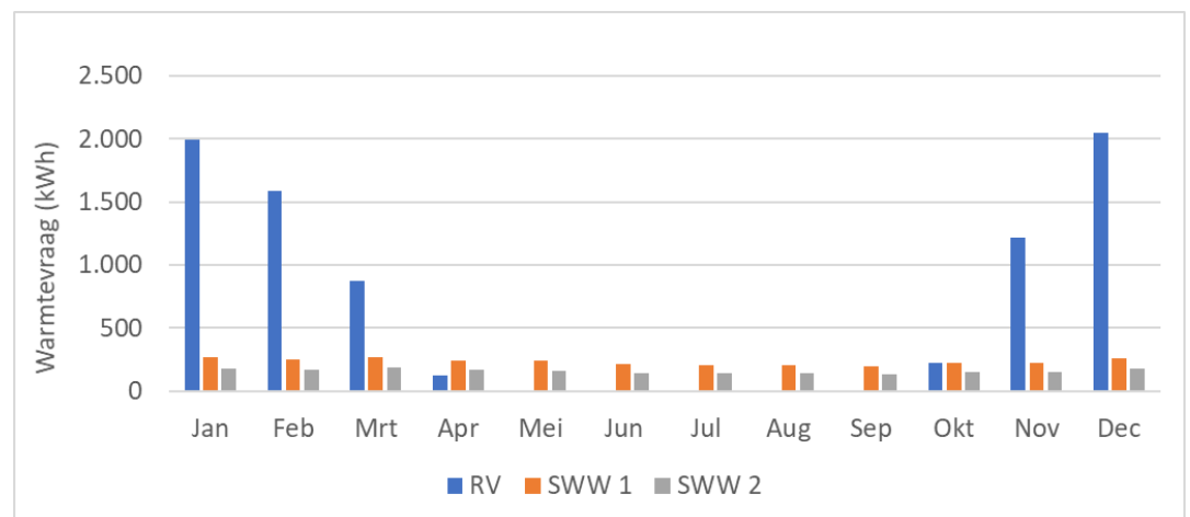
Figuur 3.1. Warmtevraagverdeling over het jaar, met in blauw de ruimteverwarmingsvraag (RV) en in oranje en grijs de twee scenario's voor sanitair warm water (SWW). Profiel over het jaar via Polysun software met weerprofiel Eindhoven.
