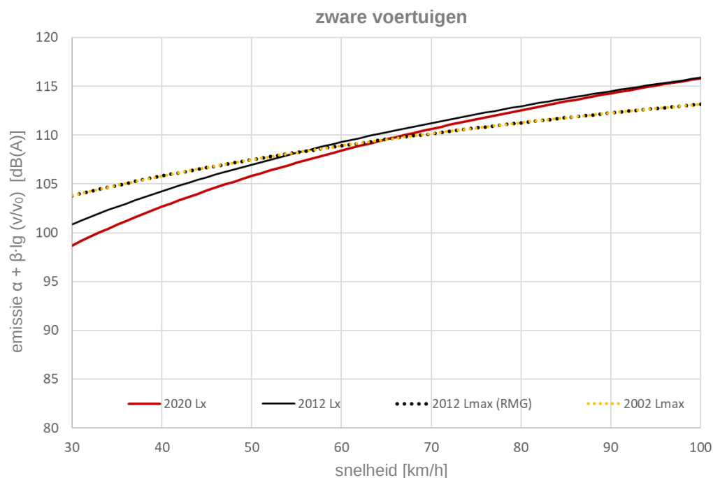
Figuur 4.3 Emissie \alpha + \beta \cdot \lg(v/v_0) in dB(A), voor zware voertuigen als functie van de snelheid. De doorgetrokken lijnen tonen de emissie die is afgeleid uit gemeten geluidexpositie-niveaus ( L_x ) van voertuigpassages in 2020 en 2012 (uit metingen 2009/2010). De gestippelde lijnen tonen de emissie die is afgeleid uit geluidniveaus L_{max} van voertuigpassages in 2002, die in het huidige Reken- en meetvoorschrift geluid 2012 is gebaseerd op de metingen van 2002.
