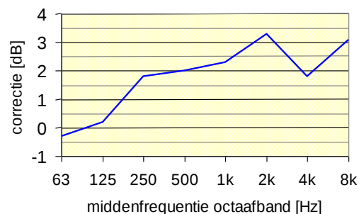
Figuur 2.2 'Empirische correctie' in de octaafbanden van 63 Hz t/m 8 kHz, variërend van 0 tot (ruim) 3 dB. De (overwegend) positieve correctie is van de emissie afgetrokken, dus de emissie is naar beneden bijgesteld.
