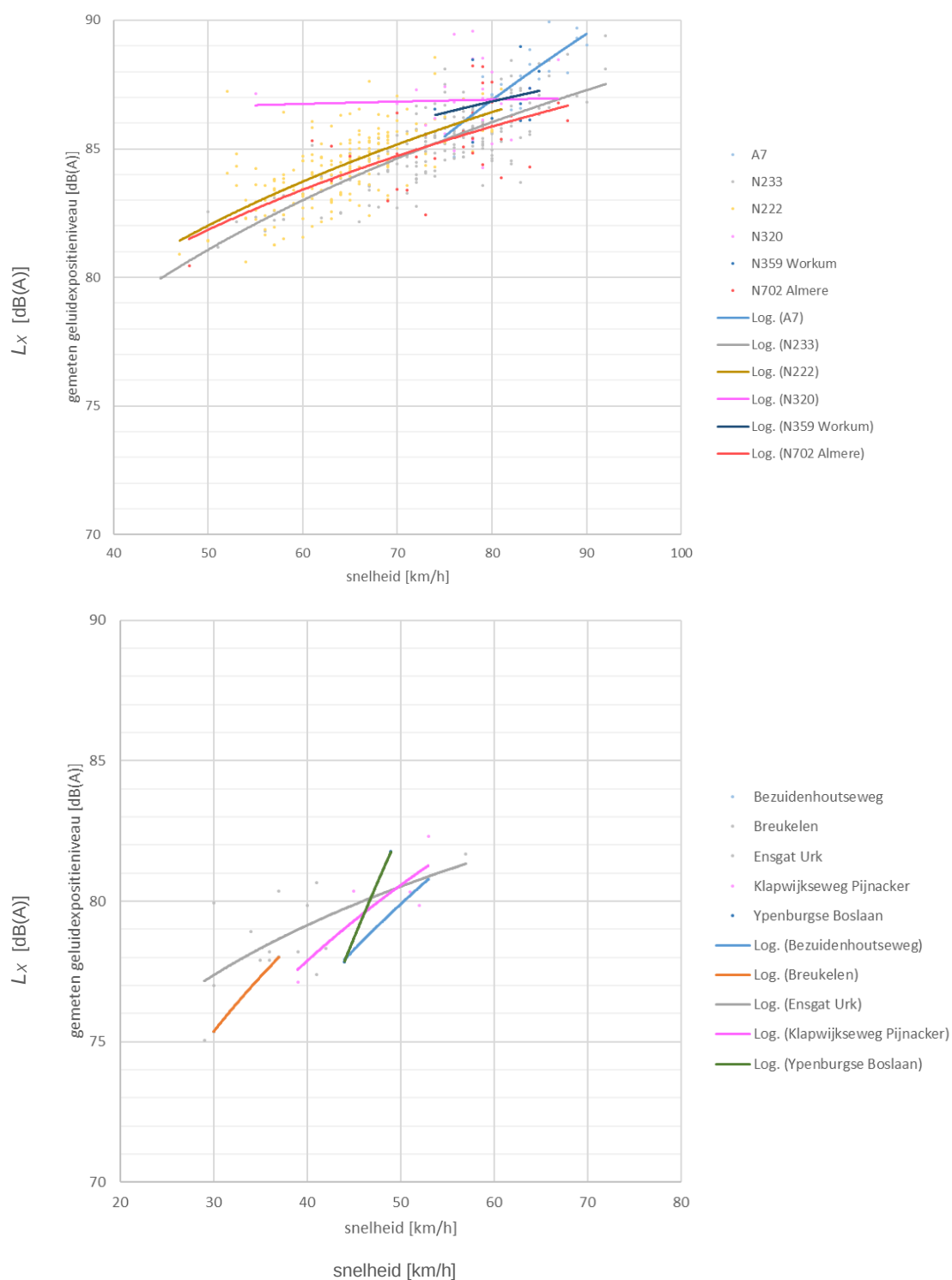
Figuur 3.4 Regressielijnen volgens L_x = A + B \cdot \lg(v/v_0) door de gemeten geluidexpositieniveaus in dB(A) per meetlocatie voor zware voertuigen , met boven de locaties met maximum snelheden vanaf 70 km/h en onder de locaties met maximum snelheden t/m 50 km/h.
