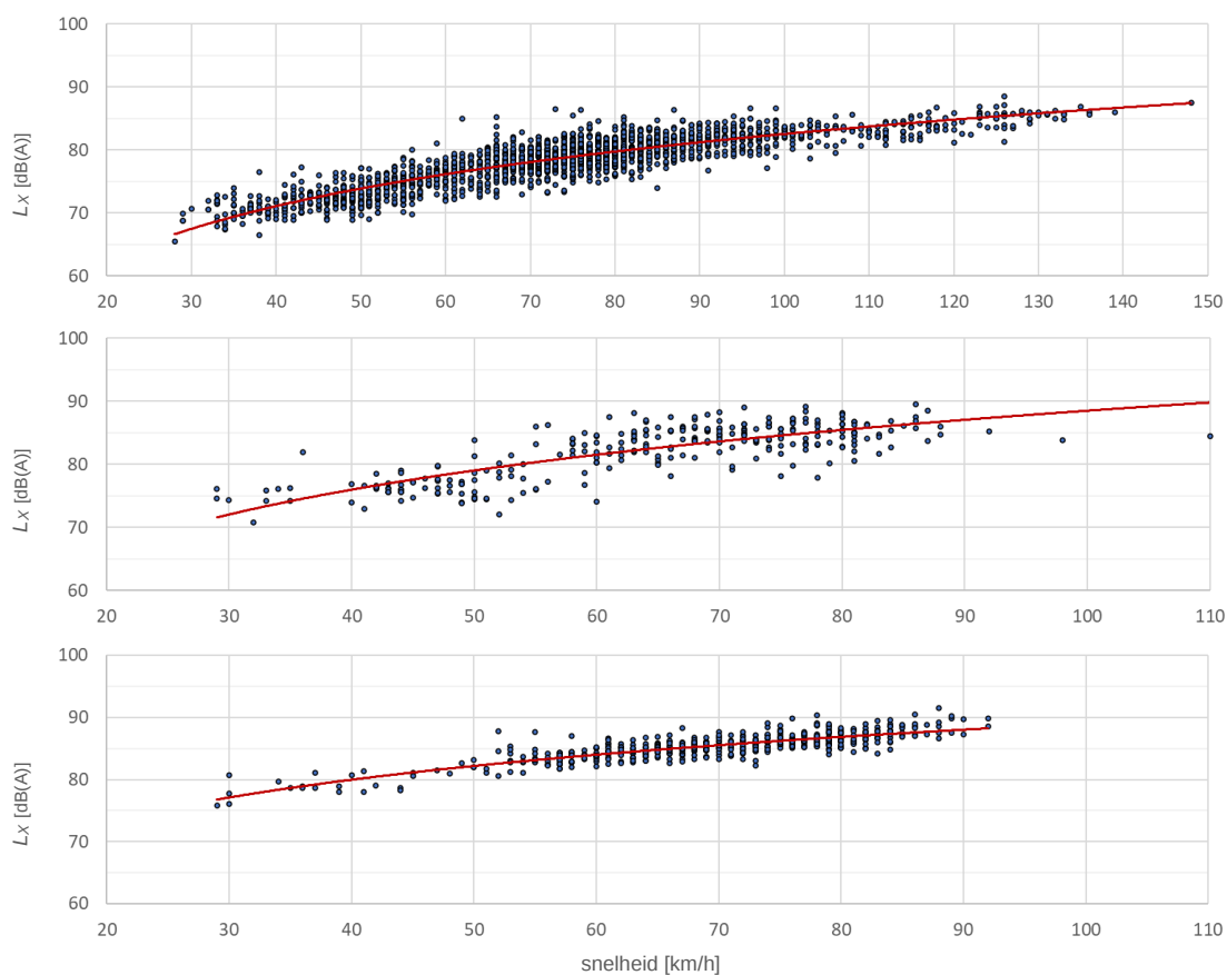
Figuur 3.1 Regressielijnen (doorgetrokken rode lijnen, volgens L_x = A + B \cdot \lg(v/v_0) ) door de gemeten geluidexpositieniveaus in dB(A) voor lichte voertuigen (boven), middelzware voertuigen (midden) en zware voertuigen (onder).
