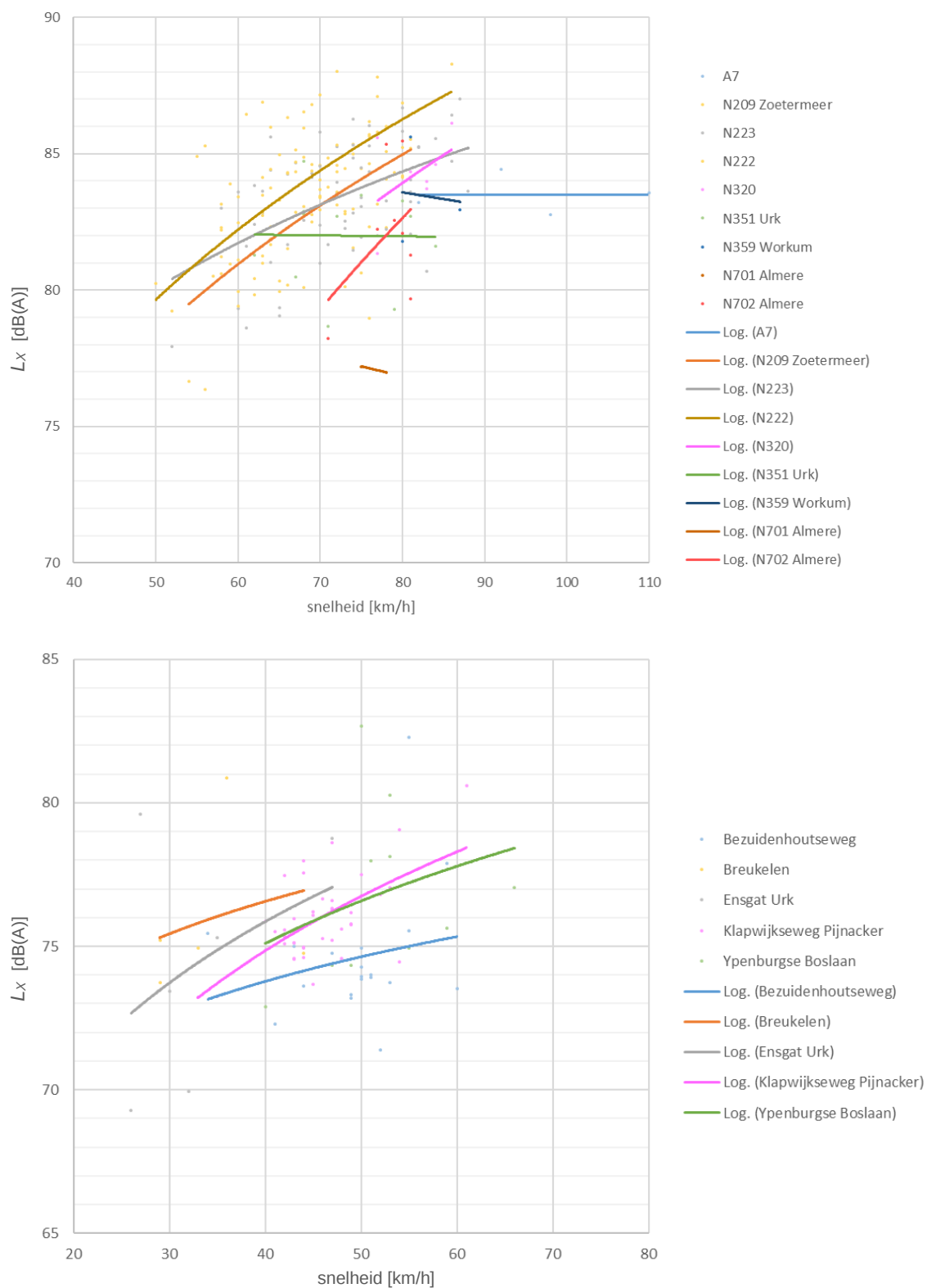
Figuur 3.3 Regressielijnen volgens L_x = A + B \cdot \lg(v/v_0) door de gemeten geluidexpositieniveaus in dB(A) per meetlocatie voor middelzware voertuigen , met boven de locaties met maximum snelheden vanaf 70 km/h en onder de locaties met maximum snelheden t/m 50 km/h.
