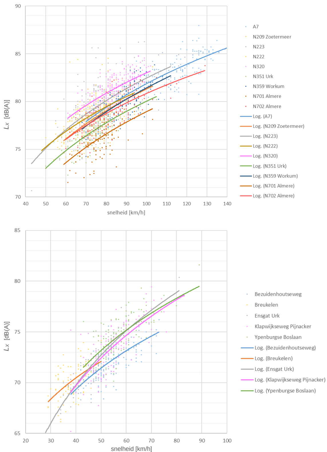
Figuur 3.2 Regressielijnen volgens L_x = A + B \cdot \lg(v/v_0) door de gemeten geluidexpositieniveaus in dB(A) per meetlocatie voor lichte voertuigen , met boven de locaties met maximum snelheden vanaf 70 km/h en onder de locaties met maximum snelheden t/m 50 km/h.
