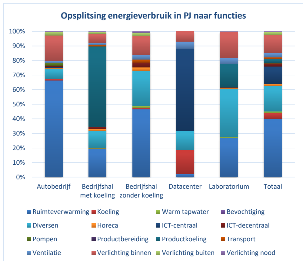
Figuur S3 Resultaat opsplitsing totaal energieverbruik (PJ) naar energiefunctie per gebouwtype
