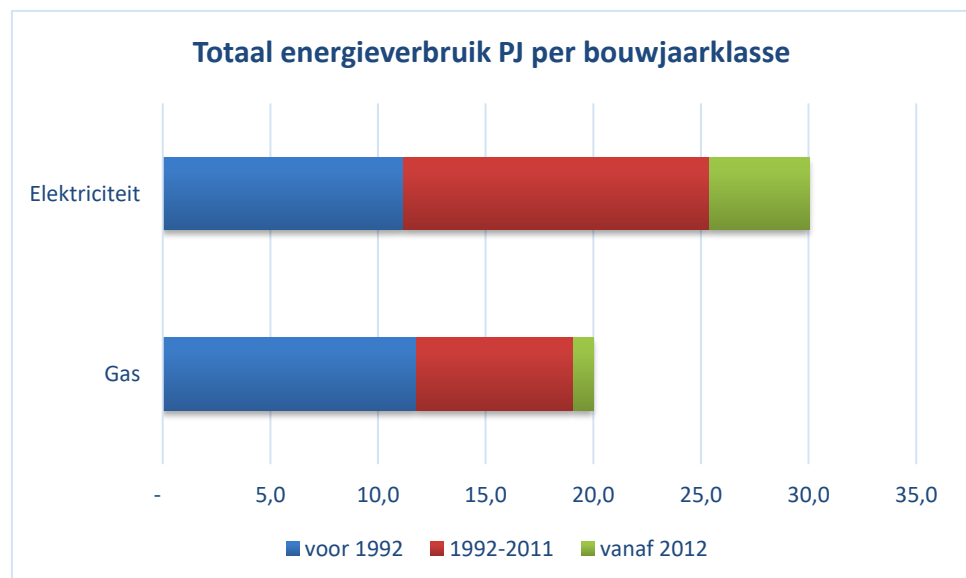
Figuur 8: Totaal bottom-up berekende energieverbruik (PJ) van bedrijfshallen onderverdeeld naar bouwjaarklasse
