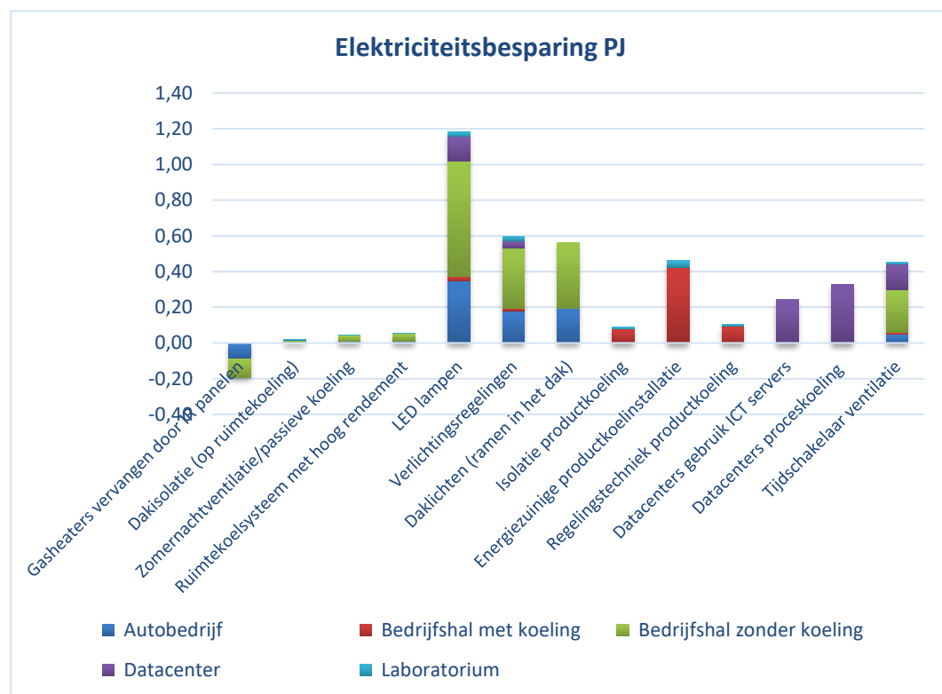
Figuur 13: Onderverdeling elektriciteitsbesparing (PJ) per maatregel naar gebouwtype
