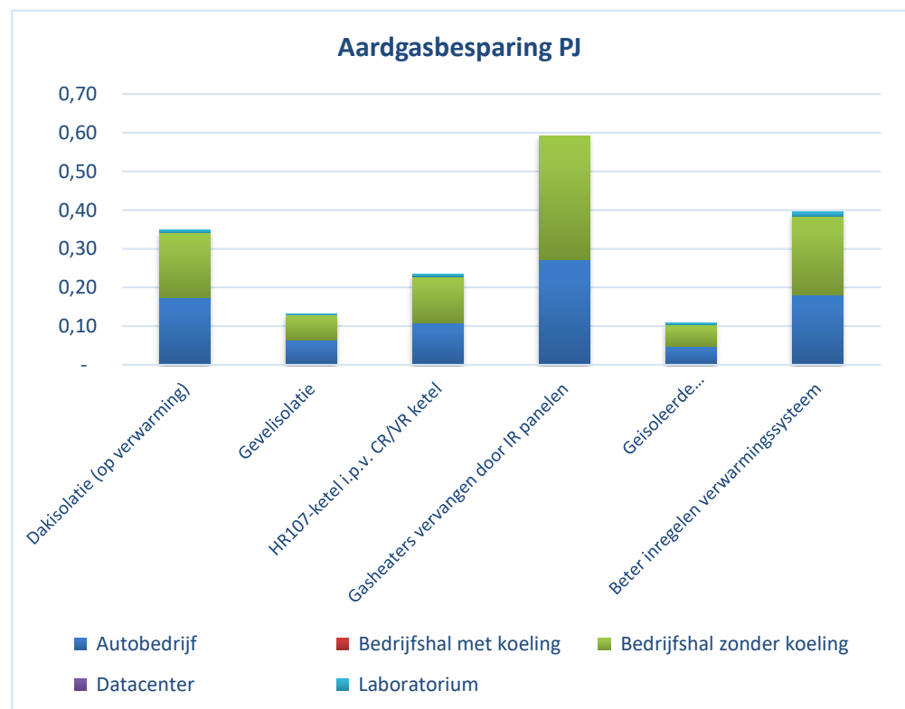
Figuur 12: Onderverdeling aardgas besparing (PJ) per maatregel naar bouwtype
