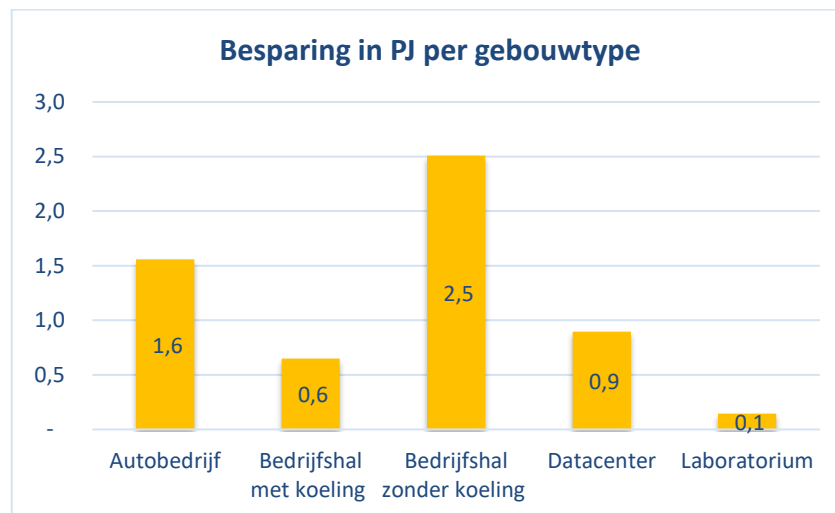
Figuur 16: Resultaat besparing (PJ) per gebouwtype
