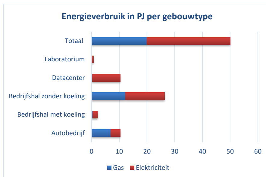
Figuur S2 Totaal bottom-up berekend energieverbruik per gebouwtype
