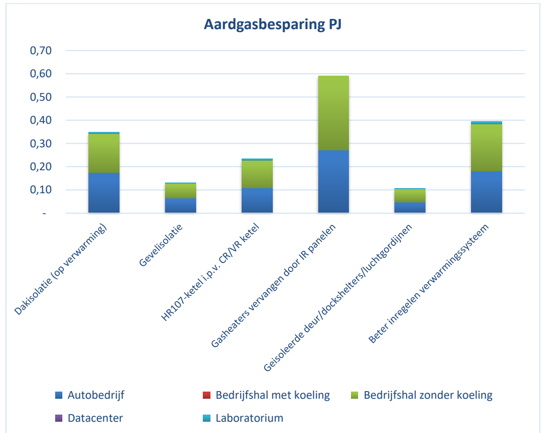
Figuur S4 Resultaat aardgasbesparing (PJ) per maatregel en per gebouwtype
