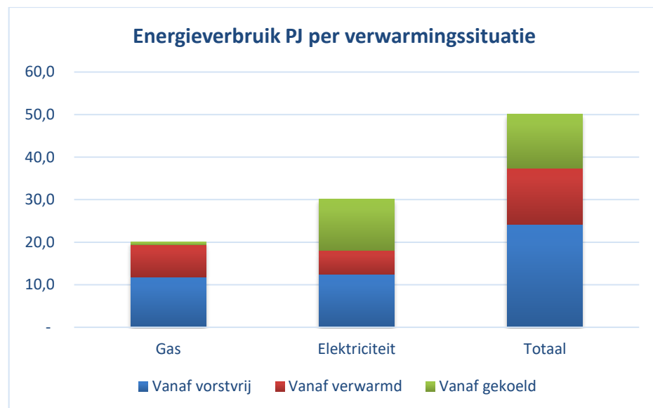
Figuur 7: Totaal bottom-up berekende energieverbruik (PJ) van bedrijfshallen met daarbij onderscheid naar verwarmingssituatie
