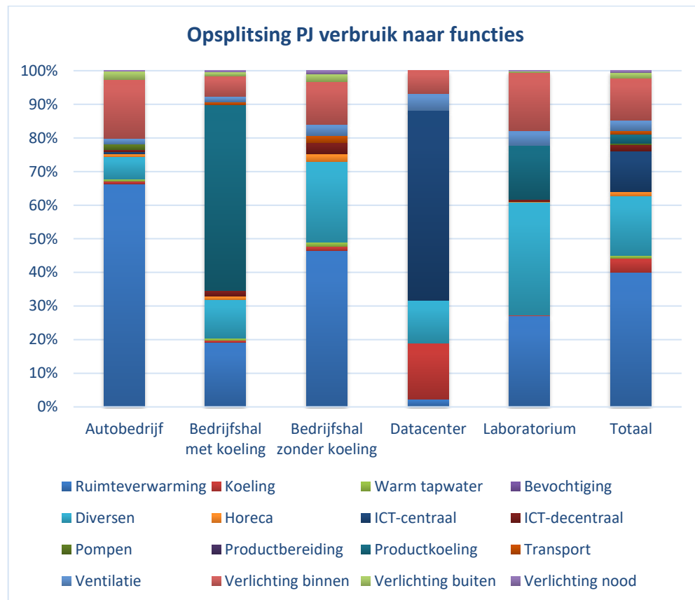
Figuur 9: Resultaat opsplitsing totaal energieverbruik (PJ) naar functie per gebouwtype
