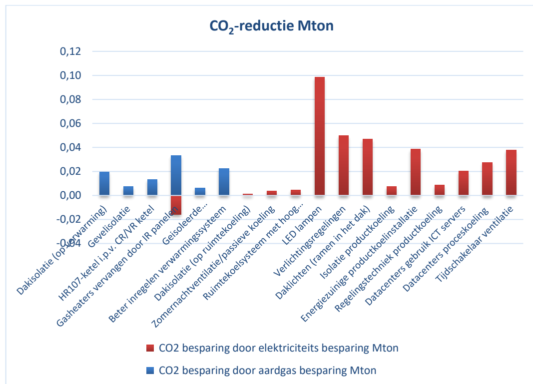
Figuur 15: CO 2 -reductie potentieel per maatregel in 2020. Exclusief hybride, all-electric warmtepompen en zon-PV
