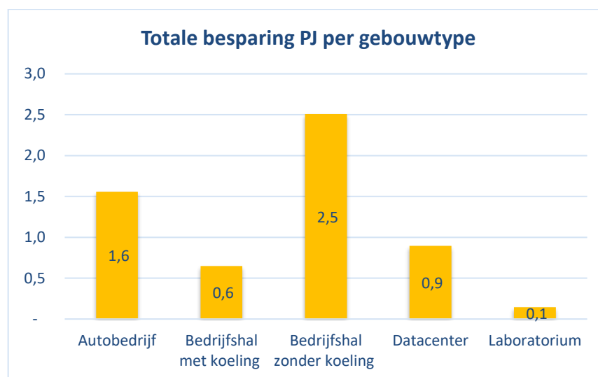
Figuur S6 Resultaat besparing (PJ) en per gebouwtype
