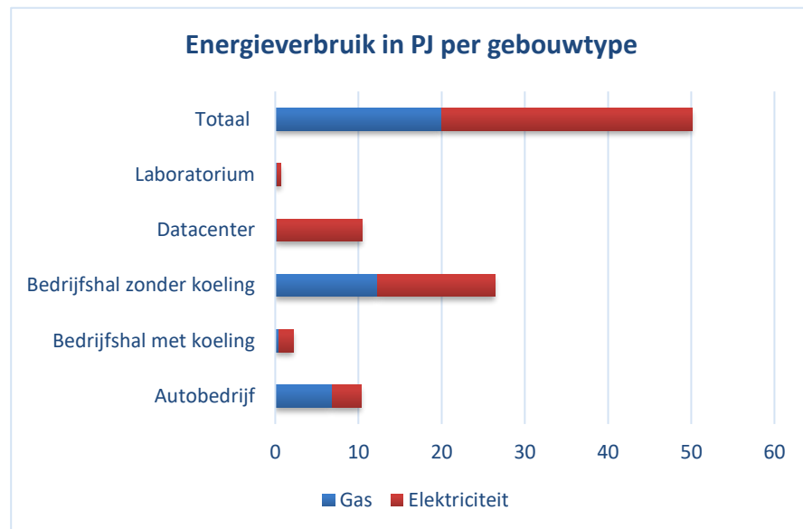
Figuur 6: Totaal bottom-up berekende energieverbruik (PJ) van bedrijfshallen met daarbij onderscheid naar gas en elektriciteit
