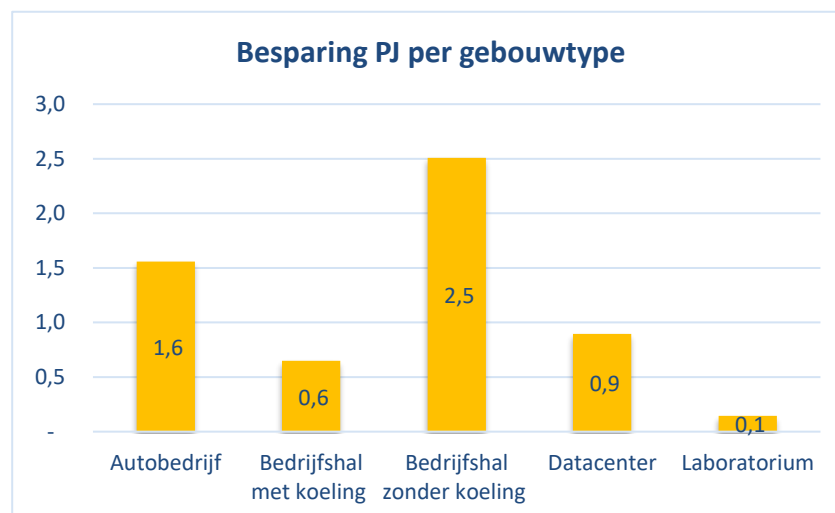
Figuur 14: Resultaat besparing (PJ) per gebouwtype
