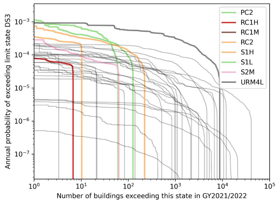
Figuur 6.4 Jaarlijkse overschrijdingskans voor schadetoestand DS2 (boven) en schadetoestand DS3 (onder) voor gasjaar 2021/2022 voor een aantal typologieën voor een koud temperatuurverloop.
