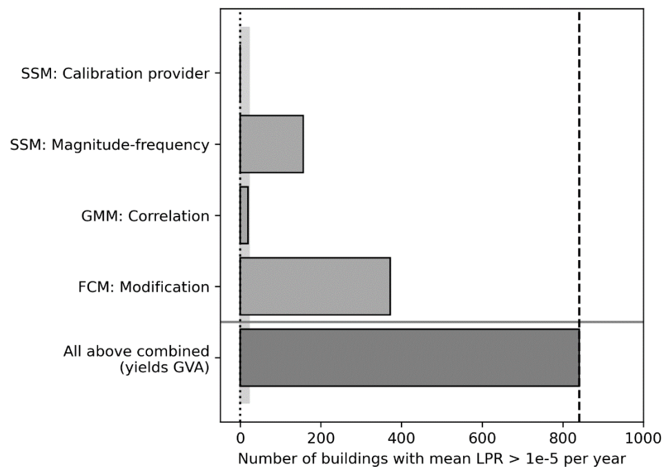
Figuur 7.3 Verskil per afzonderlijke modelkeuze (en gecombineerd) ten opzichte van SDRA 2021 in het aantal panden dat niet voldoet aan de Meijdamnorm.
