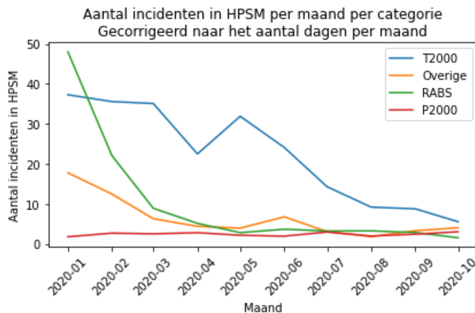
Figuur 12 Het gemiddeld aantal incidentmeldingen per dag in HPSM per categorie over de tijd. De data is gecorrigeerd naar het aantal dagen per maand in de data.
