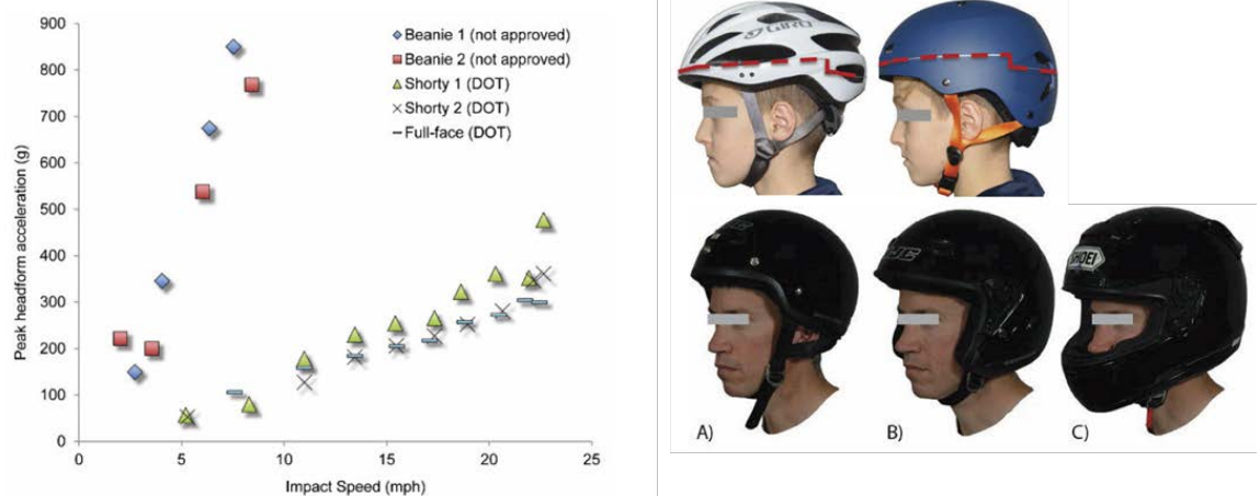
Figuur 14 Piek hoofdacceleratie voor verschillende impactsnelheden bij gebruik van verschillende typen helmen uit het onderzoek van Bonin et al [44]
