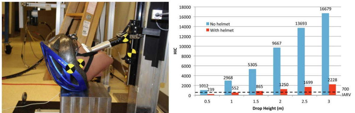
Figuur 13 Testopstelling (links) en resultaten (rechts) uit onderzoek van Crompton et al [43]
