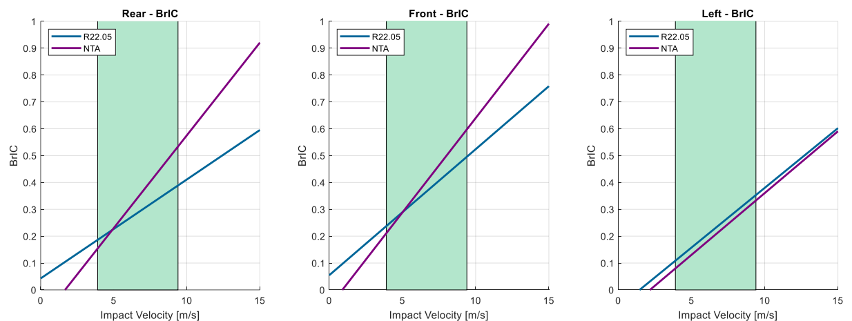
Figuur 6 Overdrachtsfuncties van impactsnelheid naar BrIC voor de, voor de drie locaties, op basis van een lineaire fit in de helmtestdata, voor bromfietshelm (R22.05) en SEPAC-helm (NTA 8776).
