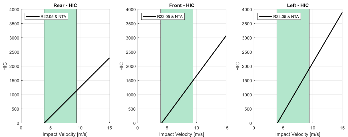
Figuur 5 Overdrachtsfuncties van impactsnelheid naar HIC15, voor de drie locaties, op basis van een lineaire fit in de helmtestdata, voor bromfietshelm (R22.05) en SEPAC-helm (NTA 8776) gecombineerd.
