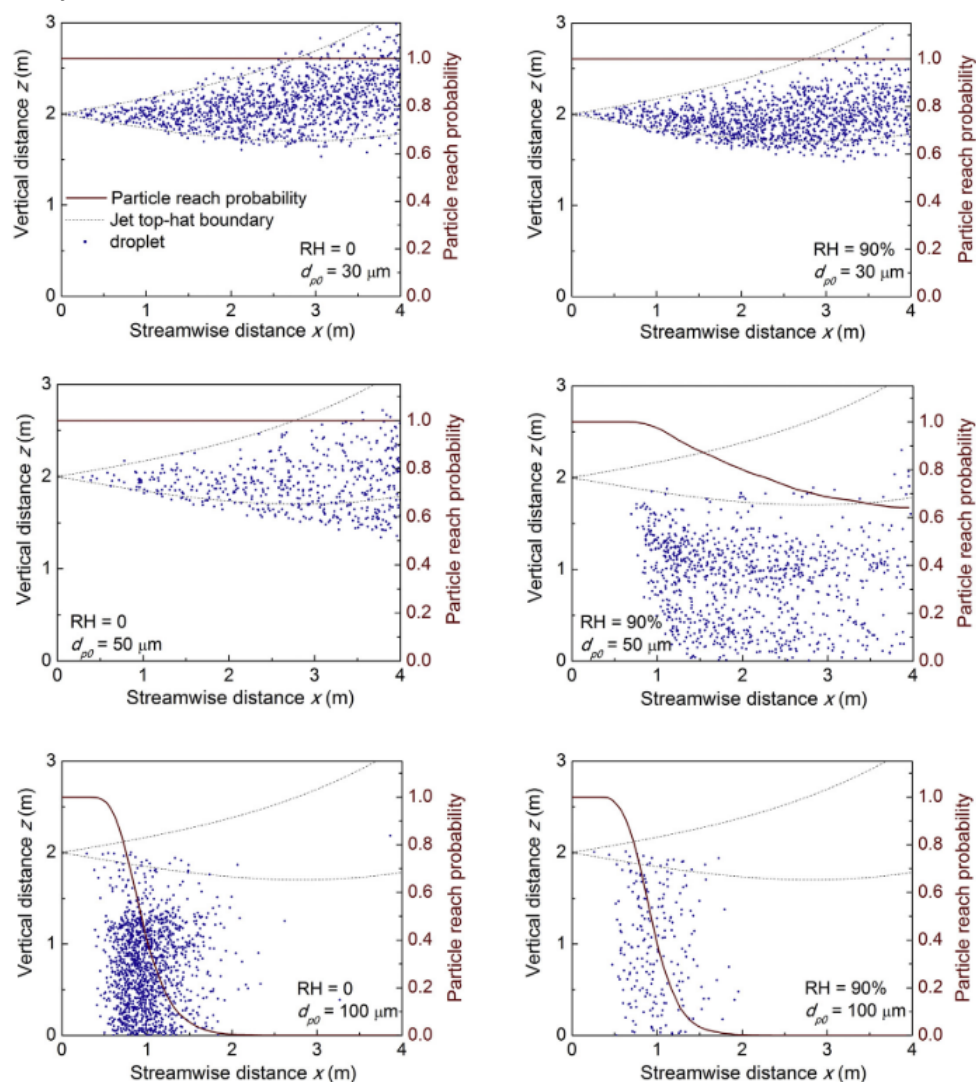
Figuur 19. Berekende horizontale afstand die drie deeltjesgroottes ( 30\text{ }\mu\text{m} , 50\text{ }\mu\text{m} , 100\text{ }\mu\text{m} ) afleggen bij het simuleren van een kuch ( t = 50\text{ s} voor 30\text{ }\mu\text{m} , t = 200\text{ s} voor 50\text{ }\mu\text{m} en 100\text{ }\mu\text{m} ). Er is in de studie rekening gehouden met verdamping, de linkerkant is gesimuleerd bij een relatieve vochtigheid van 0\% , de rechter bij 90\% . Initiële snelheid is 10\text{ m/s} (Wei & Li, 2015).
