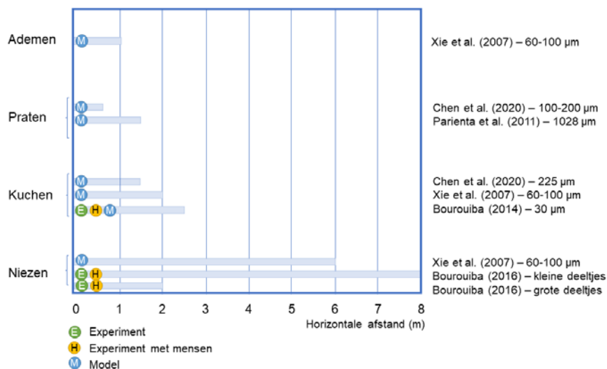
Figuur 21. Overzicht van de horizontale afstand die deeltjes >60 µm afleggen die bij meerdere studies zijn bemeten (in laboratoriumsetting) en berekend (verdamping meegenomen en zonder luchtstroming). E, experimenten; H, menselijke deelnemers; M, modelleren.
