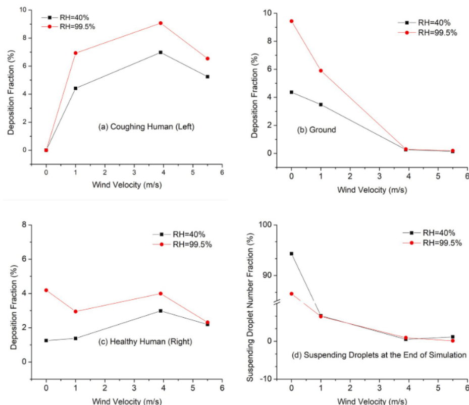
Figuur 15. Effect van luchtsnelheid en relatieve vochtigheid op druppel depositie en suspensie voor depositie fractie op de kuchende persoon (a), op de grond (b), op de gezonde persoon (c) en de druppelsuspensie als functie van de luchtsnelheid (d) (Feng et al., 2020).
