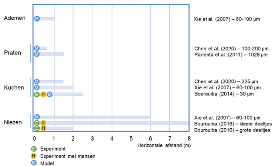
Figuur 1. Overzicht van de horizontale afstand die deeltjes >60 µm afleggen die bij meerdere studies zijn bemeten (in laboratoriumsetting) en berekend (verdamping meegenomen en zonder luchtstroming). E, experimenten; H, menselijke deelnemers; M, modelleren.
