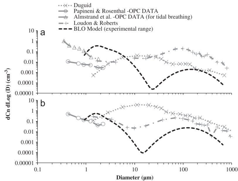
Figuur 5. Distributie deeltjesgrootte voor uitgeademde druppels bij a) praten en b) één maal kuchen (Johnson et al., 2011).
