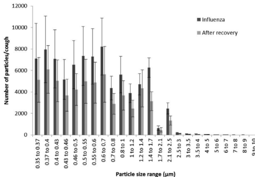
Figuur 8. Verdeling van deeltjesgroottes en hoeveelheid deeltjes die vrijkomen per kuchen bij deelnemers met influenza en nadat ze hersteld waren (Lindsley et al., 2012).
