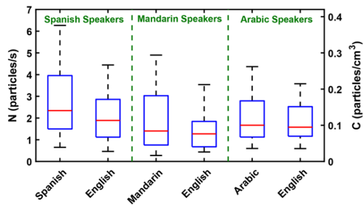
Figuur 4. Boxplot van geëmitteerde deeltjes tijdens het voorlezen van een passage tekst in twee talen (Asadi et al., 2019).
