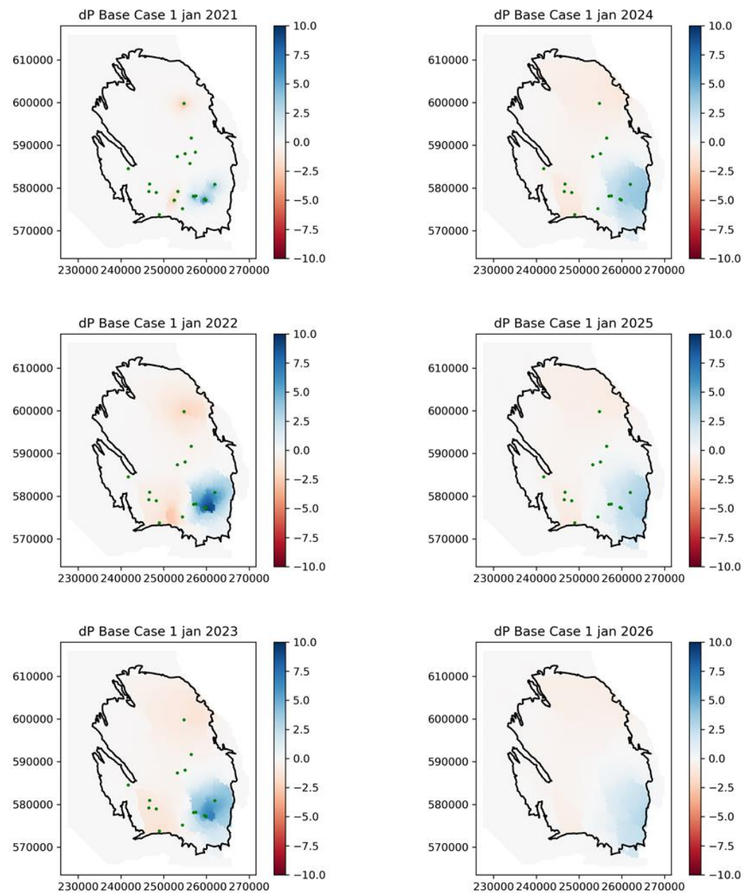
Figuur 8. Scenario Zuidooist: Jaarlijks drukverschil [in bar] ten opzichte van het referentie (BaseCase) scenario. Actieve productieclusters zijn weergegeven met groene stippen. Rood (negatief) betekent dat de reservoirdruk hoger is en blauw (positief) lager is ten opzichte van het referentie scenario.
