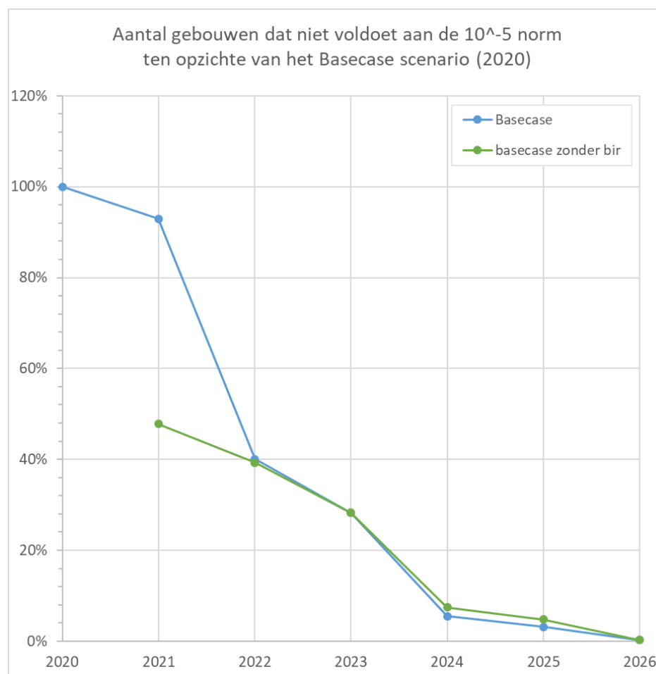
Figuur 21. Het aantal gebouwen boven de 10^{-5} risiconorm, weergegeven als percentage ten opzichte van het referentie (BaseCase) scenario in 2020. Referentie scenario weergegeven blauw, referentie scenario zonder Bierum weergegeven in groen.
