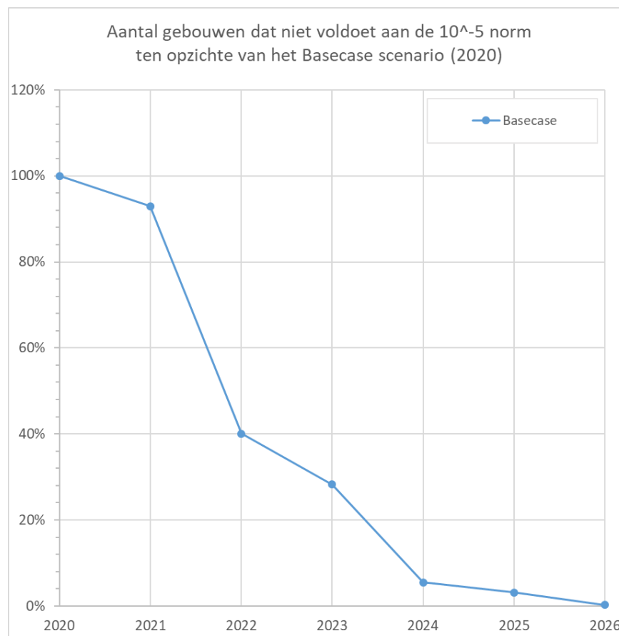
Figuur 5. Het aantal gebouwen dat niet voldoet aan de 10^{-5} risiconorm, weergegeven als percentage ten opzichte van het referentie (Basecase) scenario in 2020.
