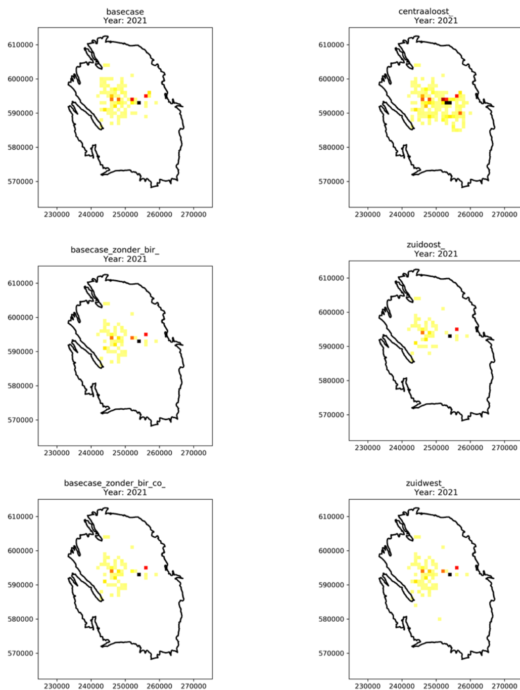
Figuur 30. Spatiële verdeling van de gebouwen die niet aan de 10^{-5} risiconorm voldoen voor alle scenario's voor het jaar 2021. Elke pixel geeft een gebied van 1 \text{ km}^2 weer. Hoe meer gebouwen zich boven de 10^{-5} risiconorm bevinden, hoe donkerder de kleur.
