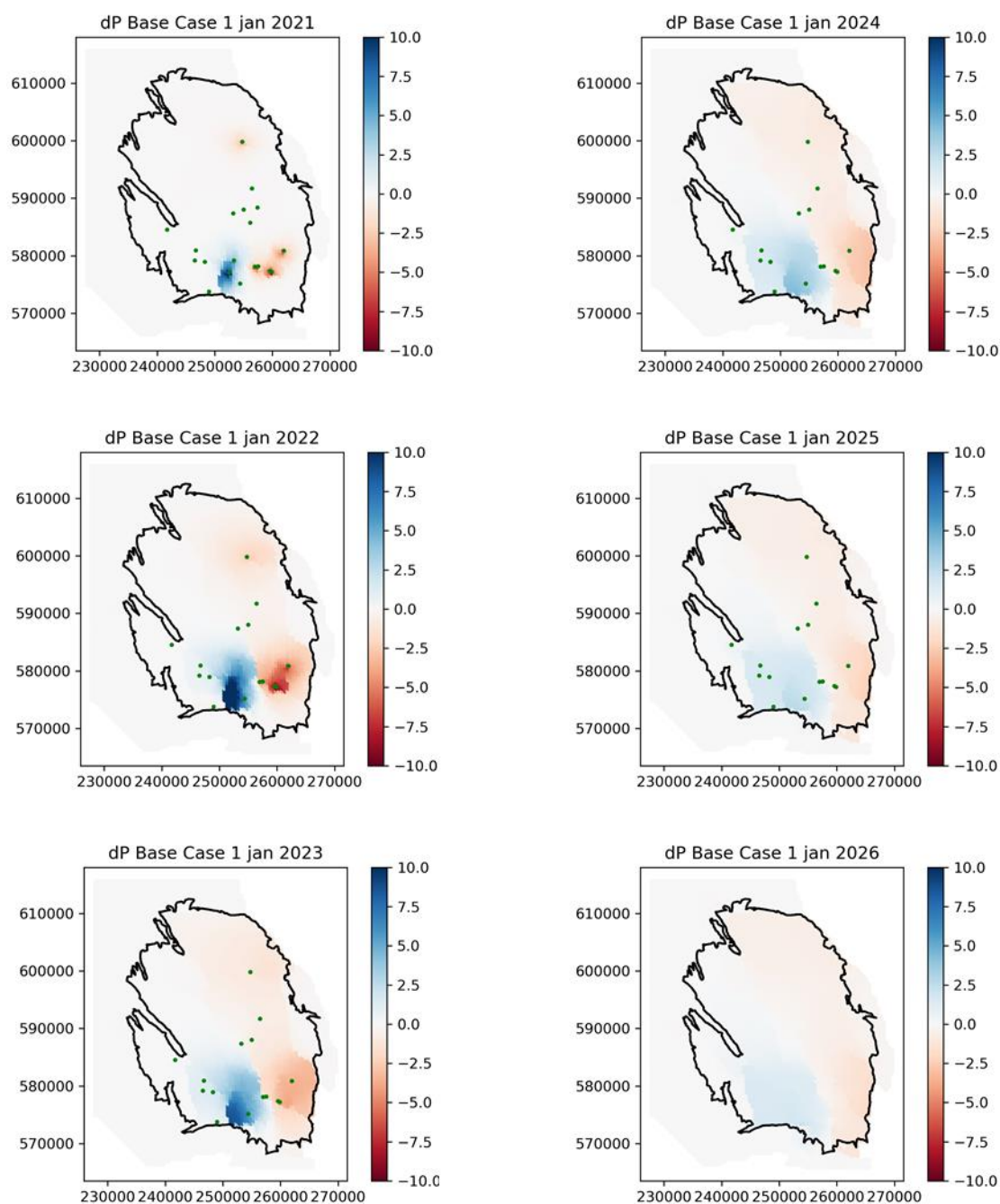
Figuur 12. Scenario Zuidwest: Jaarlijks drukverschil [in bar] ten opzichte van het referentie (BaseCase) scenario. Actieve productieclusters zijn weergegeven met groene stippen. Rood (negatief) betekent dat de reservoir druk hoger is, en blauw (positief) lager is ten opzichte van het referentie scenario.
