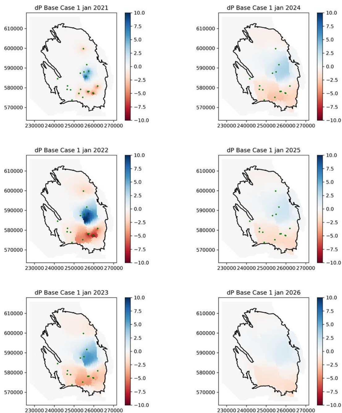
Figuur 16. Scenario Centraal-oost: Jaarlijks drukverschil [in bar] ten opzichte van het referentie (BaseCase) scenario. Actieve productieclusters zijn weergegeven met groene stippen. Rood (positief) betekent dat de reservoir druk hoger is, en blauw (negatief) lager is ten opzichte van het referentie scenario.
