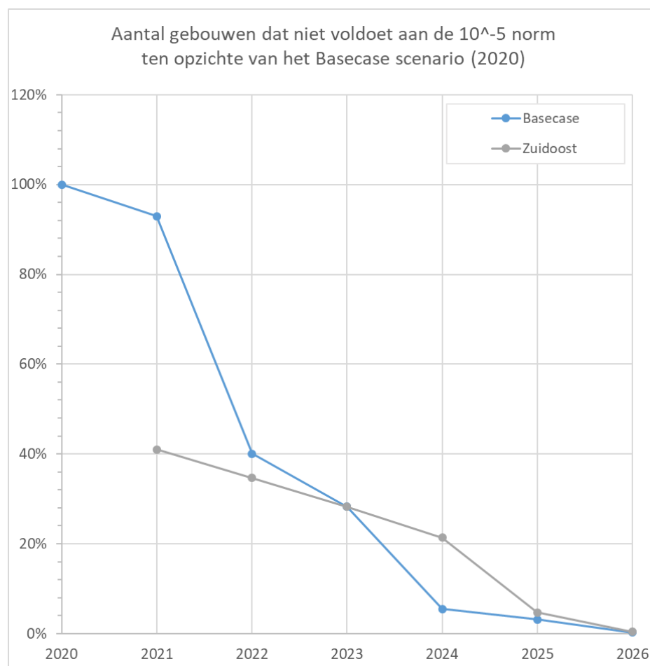
Figuur 9. Het aantal gebouwen dat niet voldoet aan de 10^{-5} risiconorm, weergegeven als percentage ten opzichte van het referentie (BaseCase) scenario in 2020. Referentie scenario weergegeven in blauw; Zuidooost scenario weergegeven in grijs.
