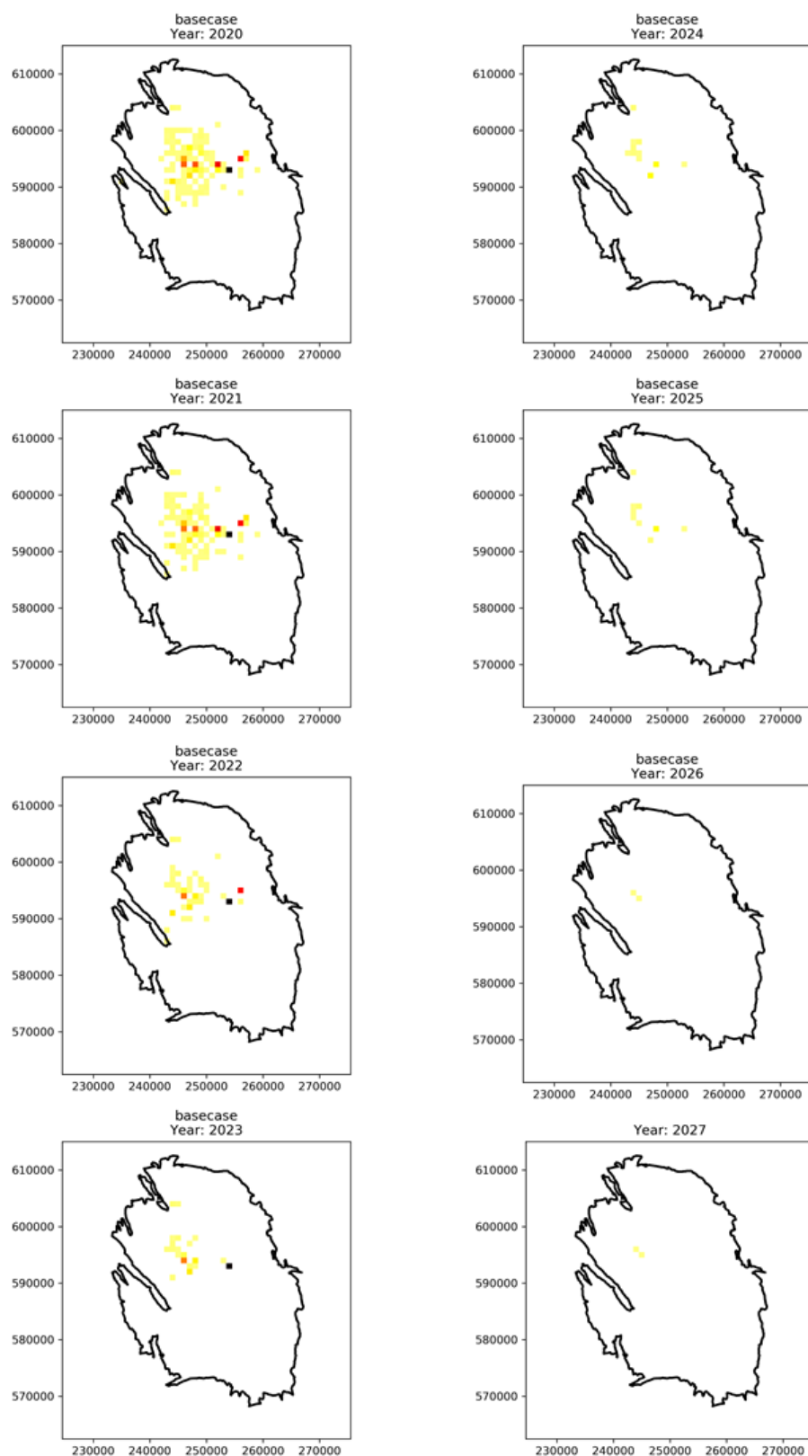
Figuur 6. Spatiële verdeling van de gebouwen die niet aan de 10^{-5} risiconorm voldoen voor het referentie (basecase) scenario. Elke pixel geeft een gebied van 1 km 2 weer. Hoe meer gebouwen zich boven de 10^{-5} risiconorm bevinden, hoe donkerder de kleur.
