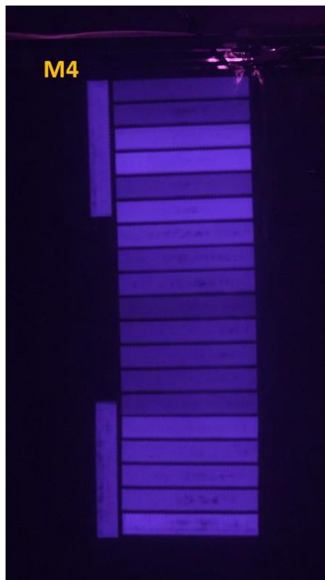
Figuur 3: Voorbeeld EL-beelden. Links: PV-halffabrikaat 'M4' heeft 1 v.d. in totaal 22 cellen niet-functionerend en is daarom afkeur. Rechts: PV-halffabrikaat 'A2' is compleet OK; de non-uniformiteit in intensiteit is gebruikelijk voor deze meettechniek.
