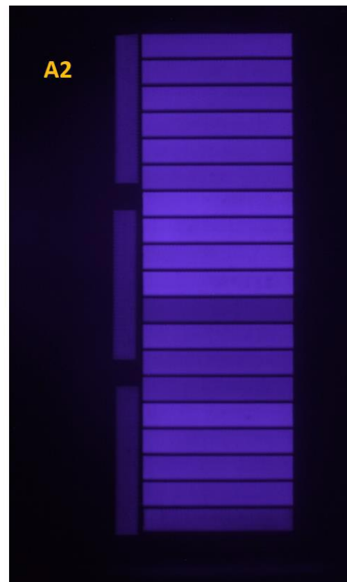
Figuur 3: Voorbeeld EL-beelden. Links: PV-halffabrikaat 'M4' heeft 1 v.d. in totaal 22 cellen niet-functionerend en is daarom afkeur. Rechts: PV-halffabrikaat 'A2' is compleet OK; de non-uniformiteit in intensiteit is gebruikelijk voor deze meettechniek.
