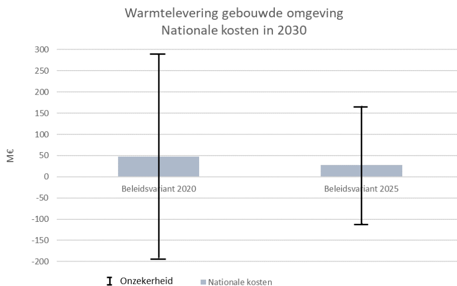
Figuur 3.1 Verandering in de nationale kosten voor warmtelevering met warmtenetten aan de gebouwde omgeving bij een mix van alternatieve warmteproductietechnologieën voor twee beleidsvarianten ten opzichte van warmtelevering met houtige biogrondstoffen
