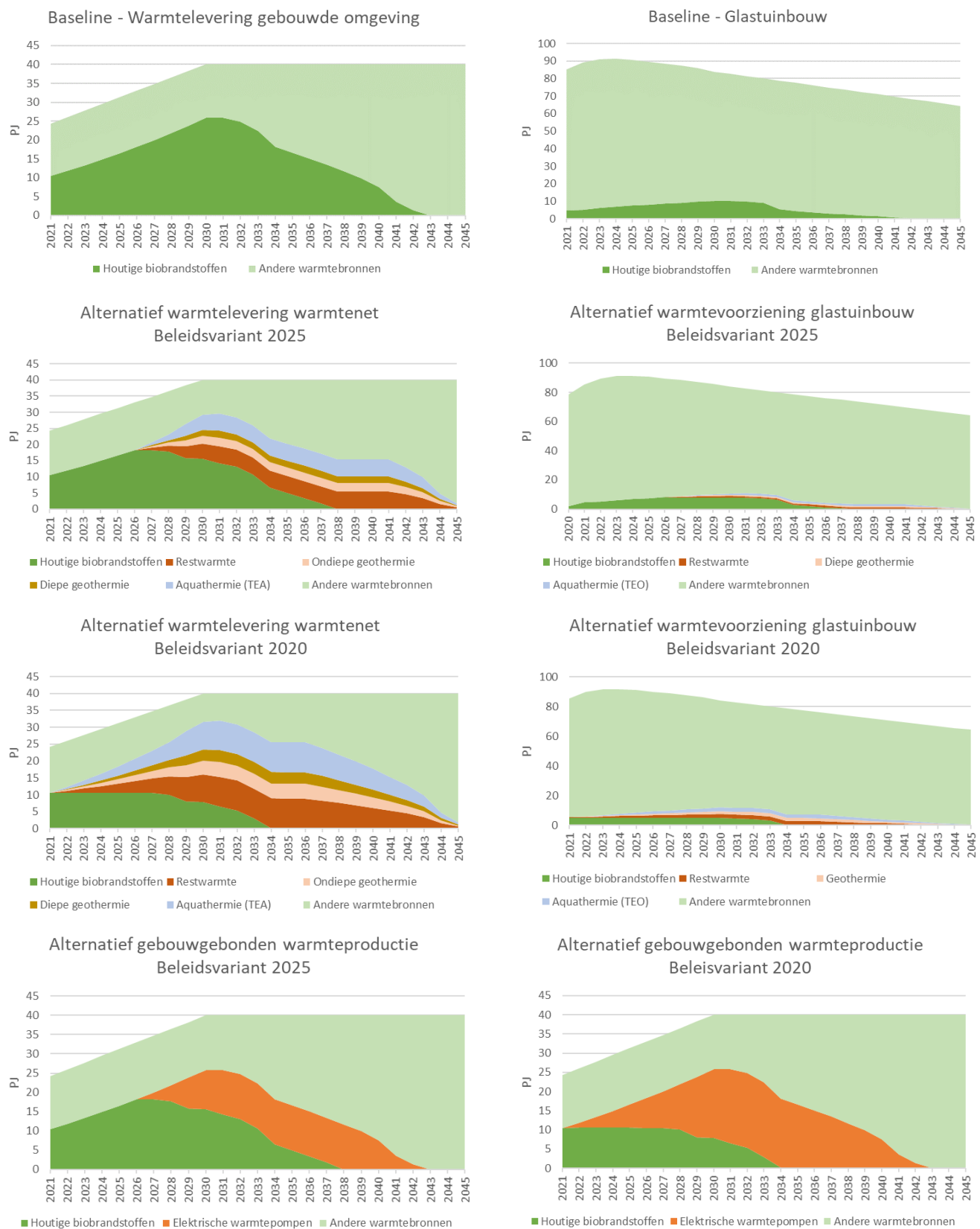
Figuur 2.1 Baseline voor warmtelevering aan gebouwde omgeving en warmteproductie in de glastuinbouw en alternatieven en beleidsvarianten. NB: Figuren geven herinvestering in duurzame warmteproductie na 2030 niet weer. In werkelijkheid zal dit wel gebeuren, waardoor de duurzame warmteproductie niet zal dalen.
