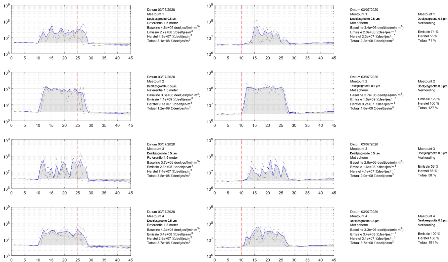
Figuur 10. Resultaten opstelling B, deeltjes \geq 0,5 \mu\text{m} . Gemeten concentraties op 4 meetpunten met resp. 1,5 meter afstand (links) en schermen (rechts). Dunne stippellijnen: drie metingen; Doorgetrokken lijn: gemiddelde daarvan. Tussen rode stippellijnen: emissieperiode.
