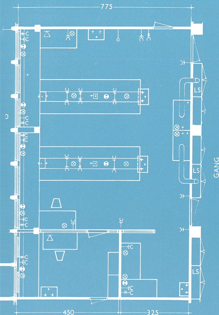
Plattegrond van een standaard laboratuureenheid
