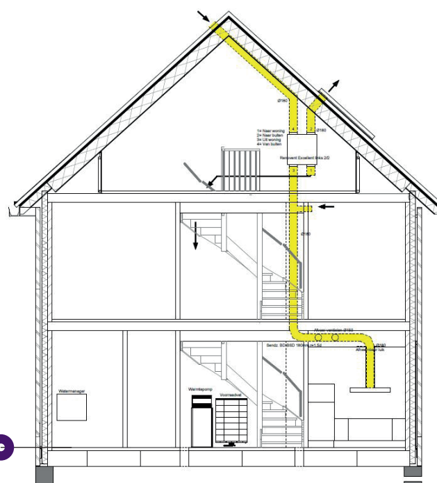
Figuur 4: Conceptueel ontwerp lucht afvoerkanaal NeroZero woning.
