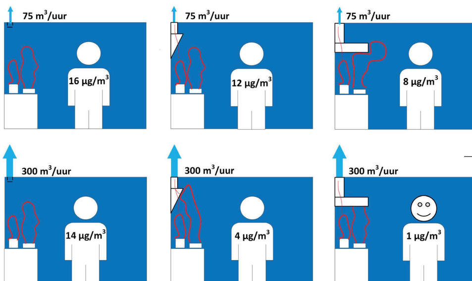
Figuur 1: Jaargemiddelde PM_{2.5} concentratieverhoging bij verblijf in woning door koken [8]. De vermelde debieten zijn de mechanische debieten tijdens het koken, na het koken is gerekend met een ventilatie + infiltratiestroom van 100 m³/uur.
