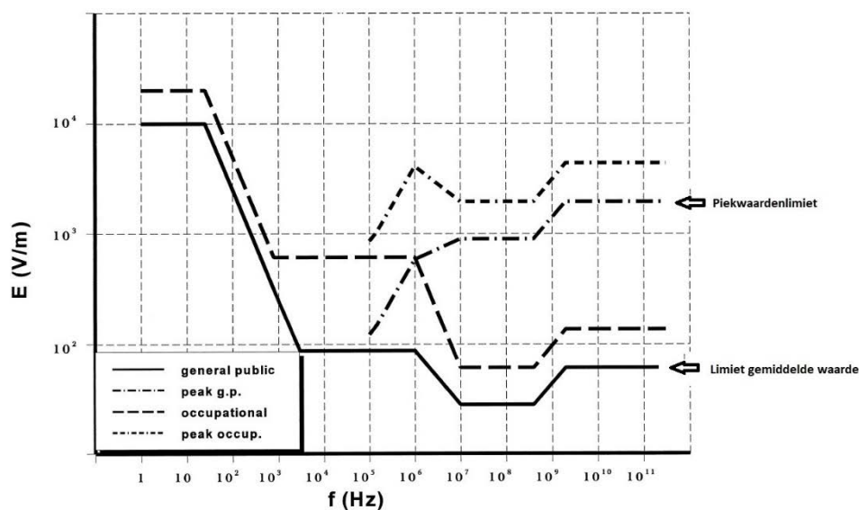
Figuur 1 Limieten voor het elektrische veld volgens ICNIRP1998. De pijlen geven de limietwaarden aan voor het algemene publiek. De bovenste pijl is de limietwaarde voor de piekveldsterkte van een gepulst signaal. De onderste pijl geeft de tijdgemiddelde veldwaarde.
