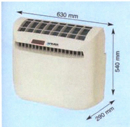
Mobile airconditioner met doorvoer door de gevel
