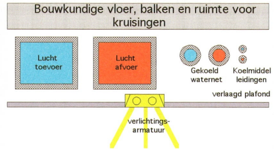
Indicatie ruimtebeslag distributiemedi: lucht, gekoeld water en koelmiddel
