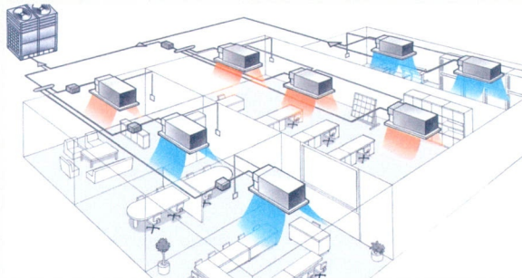
Overzicht van een VRV systeem met linksboven de centrale buitenunit (de koelmachine) en 8 binnenunits. De buitenunit staat buiten het gebouw. De binnenunits bevinden zich in de vertrekken.
