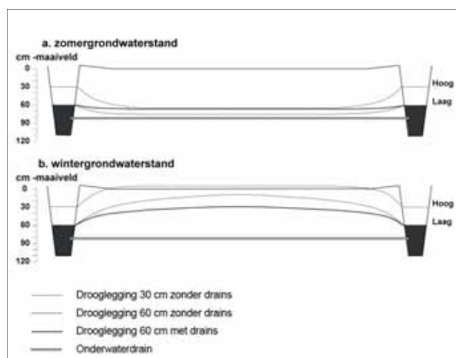
FIGUUR 2. DWARSDOORSNEDEN VAN EEN PERCEEL EN BELENDENDE SLOTTEN MET GRONDWATERSTAND (A) EN DE WINTERGRONDSTAND (B) TEN OPZICHTE VAN DE SLOOTPEILEN 30 EN 60 CM -MAAIVELD, RESP. AANGEGUID MET 'HOOG' EN 'LAAG' EN HET NIVELLERENDE EFFECT VAN ONDERWATERDRAINS (BIJ EEN SLOOTPEIL VAN 60 CM -MAAIVELD) OP DE GRONDWATERSTAND; DE ZOMER GRONDWATERSTAND WORDT VERHOOGD (TOT CIRCA GRONDWATERSTAND BIJ HOOG PEIL) EN DE WINTERGRONDWATERSTAND WORDT VERLAAGD. BRON: WOESTENBURG, 2009.
