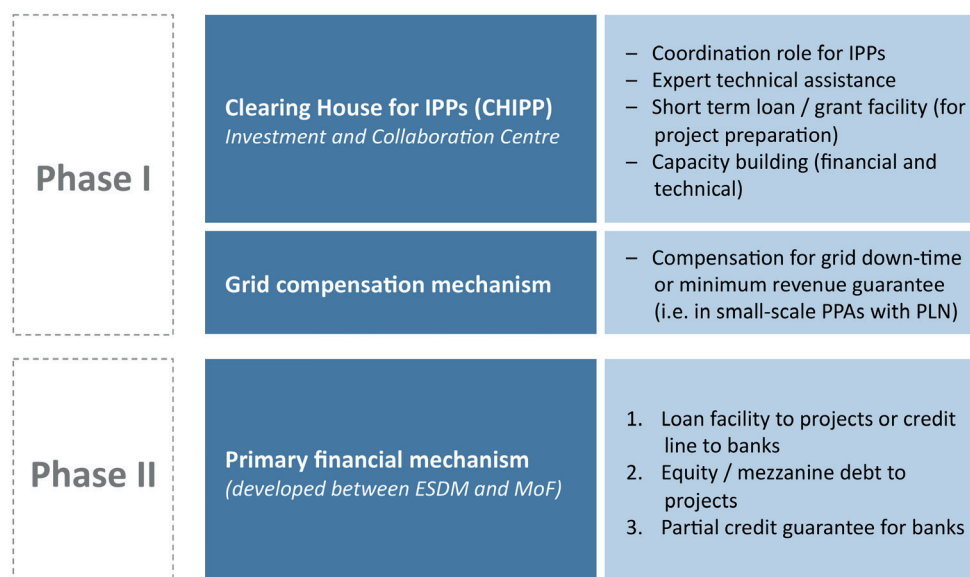
Gambar X1: Komponen-komponen NAMA
