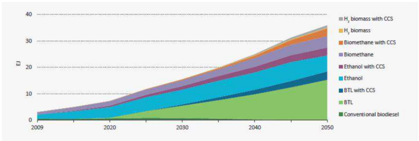
Figuur C-3 Brandstofproductie (incl. waterstof en biomethaan) uit biomassa per technologie (Bron: 2DS scenario, IEA, 2012).
