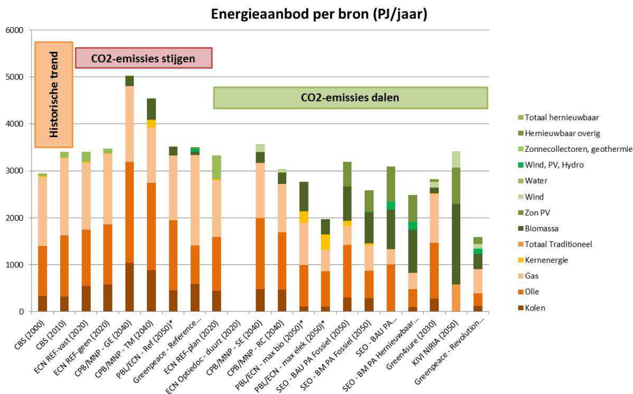
Figuur 3.7 Energieaanbod naar energiebron (PJ) in Nederlandse toekomstscenario's
