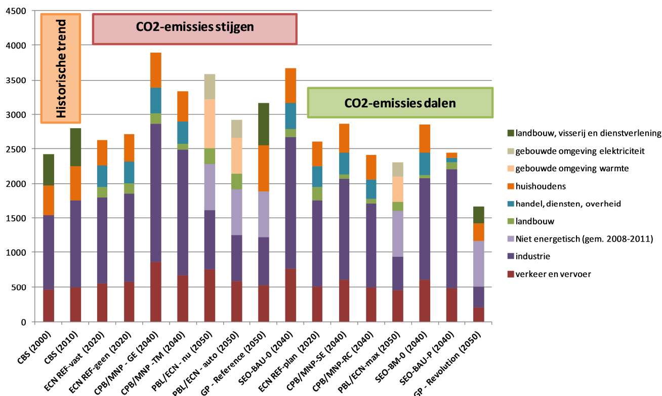
Figuur 3.6 Energievraag per sector (PJ) in Nederlandse toekomstscenario's. Indien een studie de niet-energetisch energievraag in de industrie buiten beschouwing heeft gelaten, is ter referentie het gemiddelde van de niet-energetische energievraag in de jaren 2008-2011 toegevoegd.
