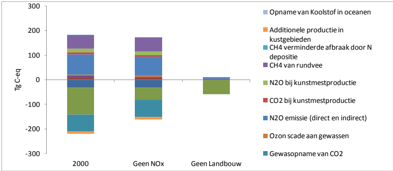
Figuur 6. De directe en indirecte effecten van totaal Nr op de koolstofbalans in Europa (Tg) voor 2000, bij het uitsluiten van landbouw en bij het uitsluiten van NOx.
