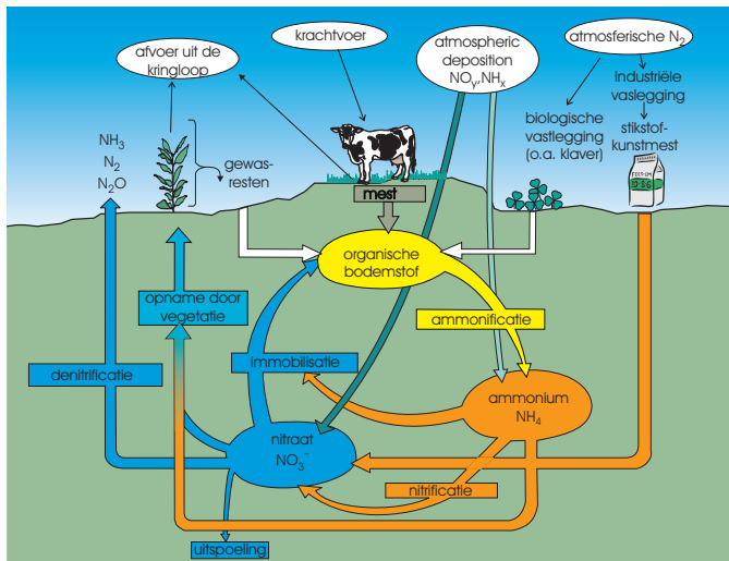
Figuur 2. De stikstofcyclus
