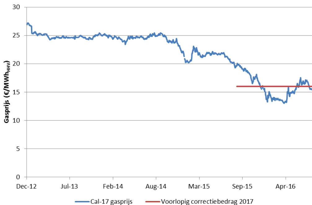
Figuur 2: Ontwikkeling van de aardgasprijs (termijnprijs voor levering in 2017) (Bron: ENDEX/ICE)
