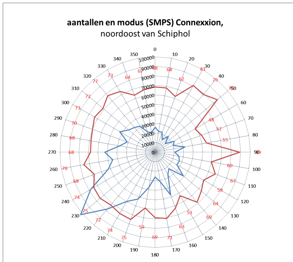
Figuur 32: Windrichtingsafhankelijke aantallen concentraties (cm -3 ) en modus (SMPS) op Nieuwe Meer/Schiphol Noord (30 apr-8 jun; 935 uur)
