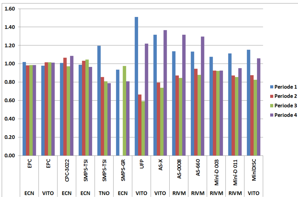
Figuur 6: Verhoudingsfactoren na toepassing van de correctiealgoritmes
