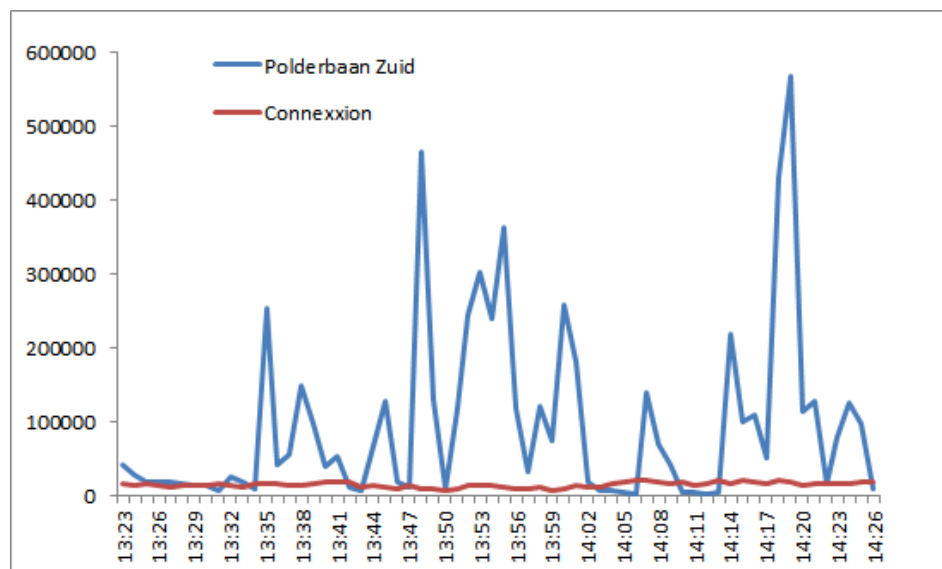
Figuur 21: Achtergrond bij Nieuwe Meer/Schiphol Noord ten opzichte van meting van de zuidkop van de Polderbaan (belast, \text{cm}^{-3} )
