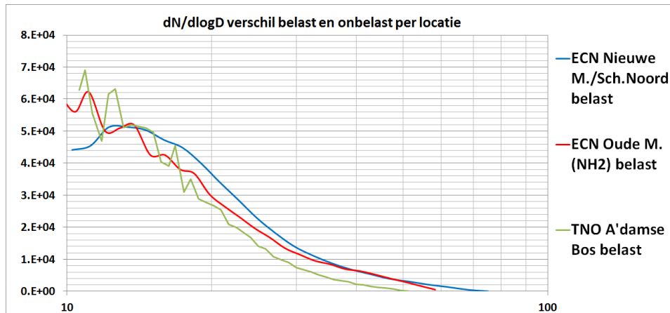
Figuur 40: Netto verschil van de spectra 'belast' en 'onbelast' per locatie
