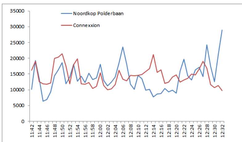
Figuur 19: Achtergrondmeting bij Nieuwe Meer/Schiphol Noord (hier aangeduid met Connexxion) vergeleken met meting op Noordkop Polderbaan (eenheid: cm -3 )
