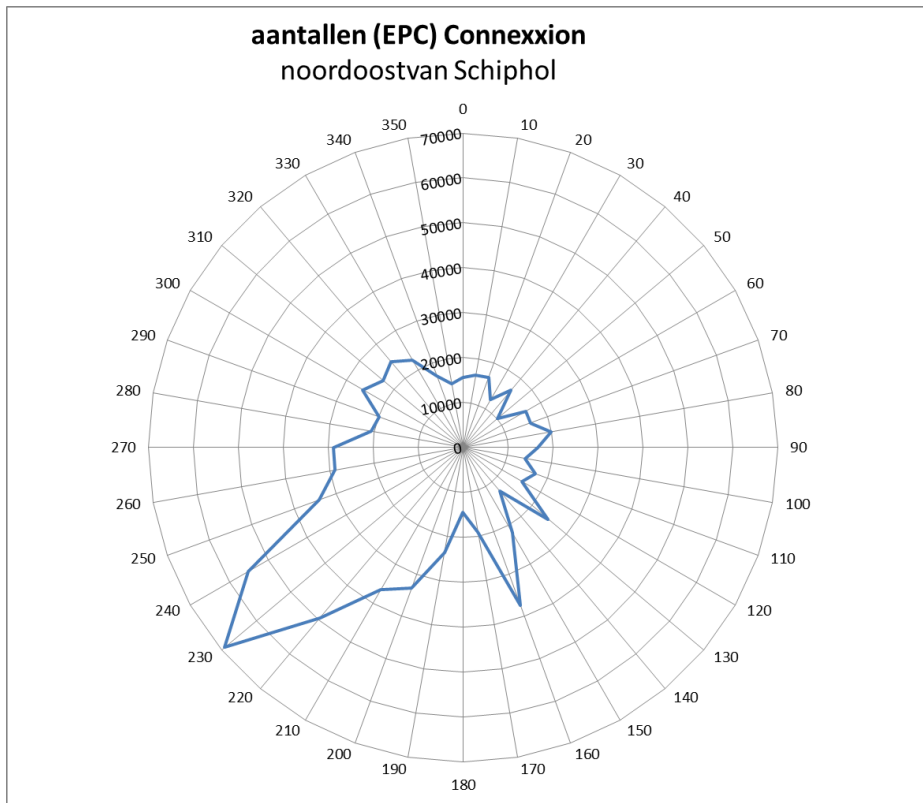
Figuur 31: Windrichtingsafhankelijke aantallenconcentraties ( \text{cm}^{-3} ) Nieuwe Meer/Schiphol Noord (30 apr-8 jun; 885 uur)
