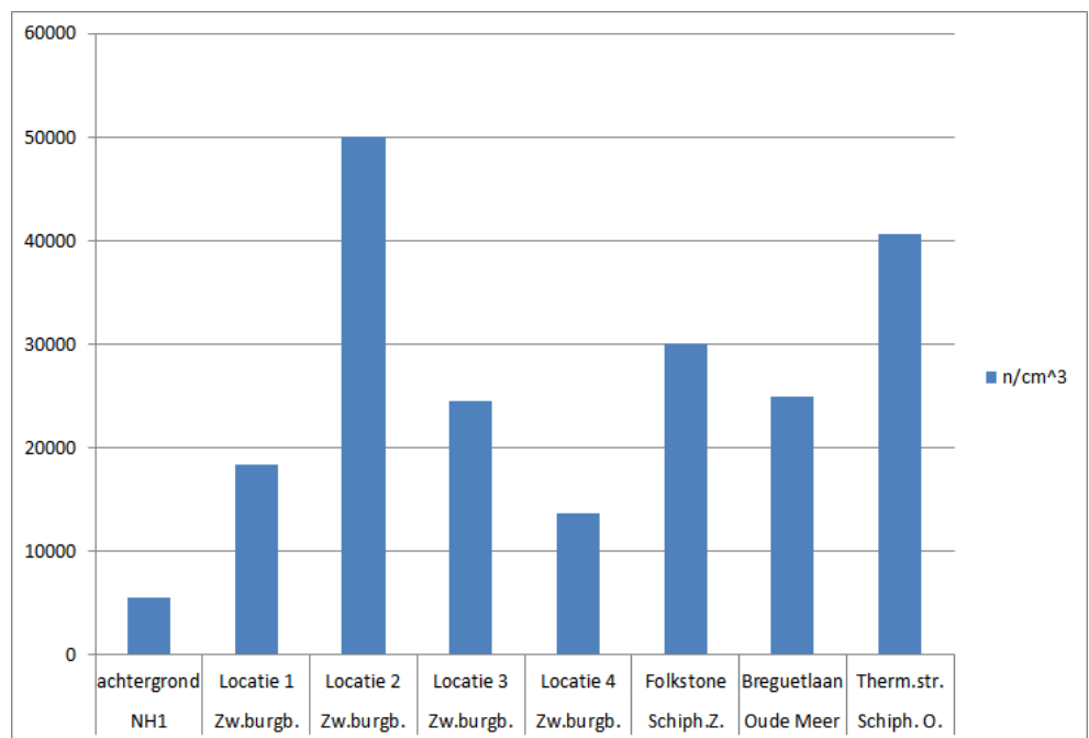
Figuur 11: Gemiddelde deeltjesconcentraties ( \text{cm}^{-3} ) op verschillende locaties rondom Schiphol tijdens de metingen op 13 april 2015
