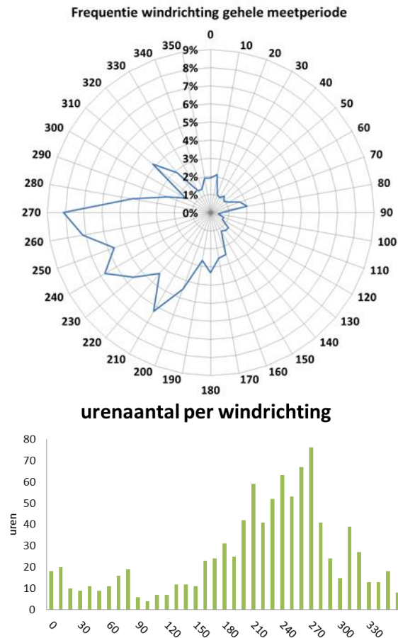
Figuur 29: Voorkomen van windrichting tijdens Fase 2 relatief (boven) en absoluut (beneden)
