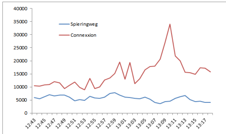
Figuur 20: Achtergrond bij Nieuwe Meer/Schiphol Noord t.o.v. meting noordkop Polderbaan, nu noord van A9 ( \text{cm}^{-3} )
