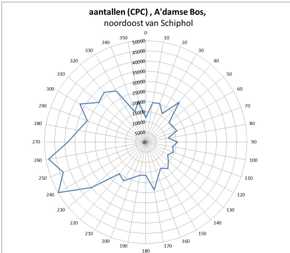
Figuur 33: Windrichtingsafhankelijke aantallenconcentraties ( \text{cm}^{-3} ) op meetlocatie Amsterdamse Bos (28 apr-28 mei; 696 uur)
