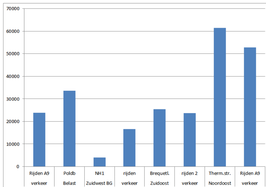
Figuur 14: De gemiddelde deeltjesconcentraties per locatie of per gereden route ( \text{cm}^{-3} )
