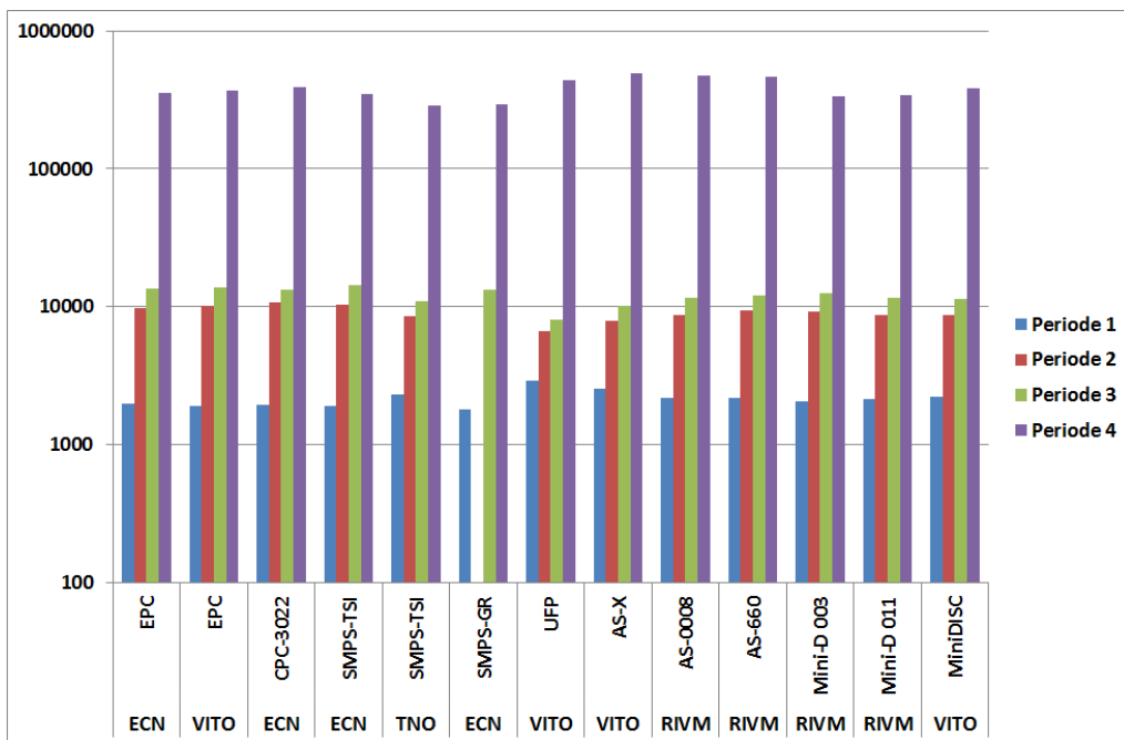
Figuur 5: Aantallenconcentraties na toepassing van de correctiealgoritmes (cm -3 )
