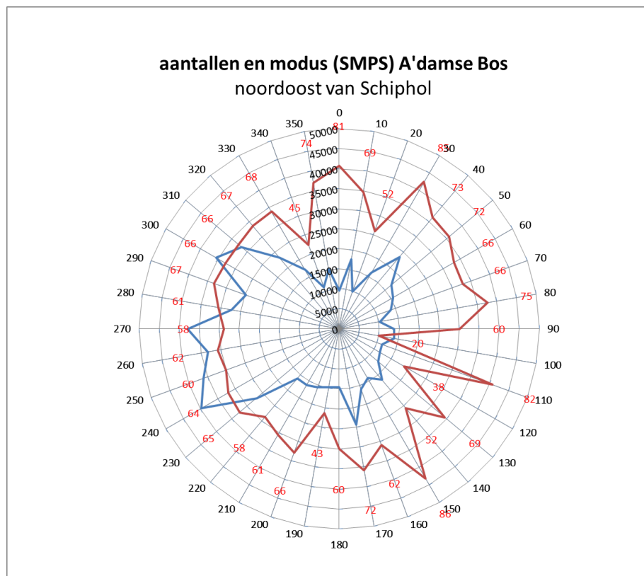
Figuur 34: Windrichtingsafhankelijke aantallenconcentraties ( \text{cm}^{-3} ) en modus (SMPS) op Nieuwe Meer/Schiphol Noord (28 apr-28 mei; 427uur)
