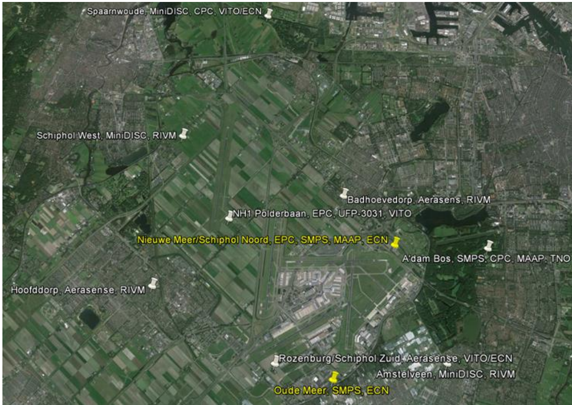
Figuur 1: Locaties van de vaste meetstations (Fase 2) in de regio Schiphol
