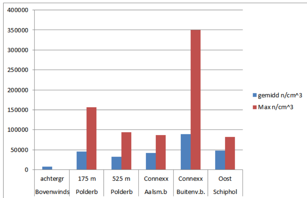
Figuur 13: De gemiddelde en maximaal gemeten aantallen ( \text{cm}^{-3} ; minuutgemiddelden) op de verschillende locaties op 14 april 2015
