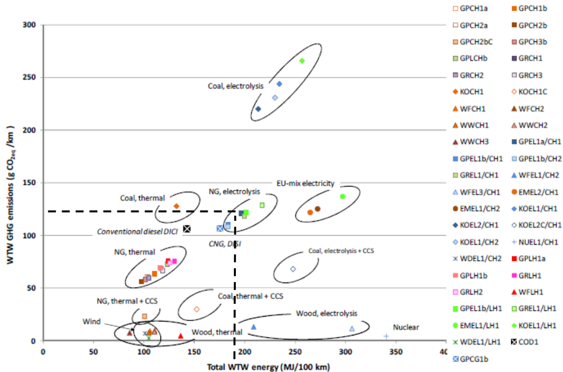
Figure 1 WTW energieverbruik en broeikasgasemissies voor 2020+ brandstofcelauto's en diverse waterstofketens (bron: JEC Well-to-Wheels analysis, Well-to-Wheels Report Version 4.a)
