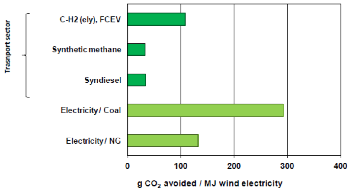
Figure 6 Indicatie van potentieel voor vermijding van CO 2 emissies via diverse alternatieven voor inzet van wind-elektriciteit (bron: JEC Well-to-Wheels analysis, Well-to-Wheels Report Version 4.a)
