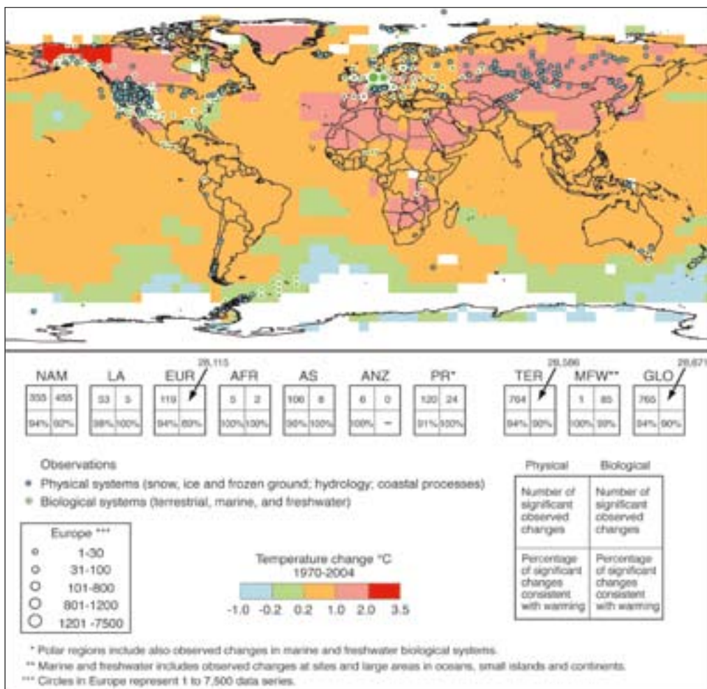
Figuur 2.1 Locaties van waargenomen veranderingen in fysische systemen (cryosfeer, hydrologie en kust) en biologische systemen (terrestrisch, marien, zoetwater), voor studies eindigend in 1990 of later met minstens twintig jaar resultaten, en temperatuurveranderingen in de periode 1970-2004. Resultaten uit 75 studies (waarvan zeventig nieuwe studies sinds het vorige IPCC-rapport (2001)) met meer dan 29.000 gegevensbestanden zijn verwerkt. Witte gridcellen: onvoldoende waarnemingen. De vierkanten bevatten gegevens voor i) regio's: NAM Noord-Amerika, SAM Zuid-Amerika, EUR Europa, AFR Afrika, AS Azië, AUS Australië, PR Polaire gebieden, en ii) TER terrestrische, mariene en zoetwater systemen (MFW), mondiale veranderingen in fysische en biologische systemen.
