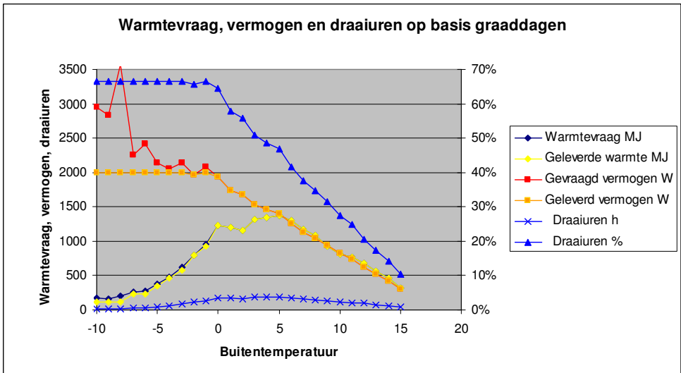
Figuur.2: Voorbeeld van gesimuleerde warmteproductie
