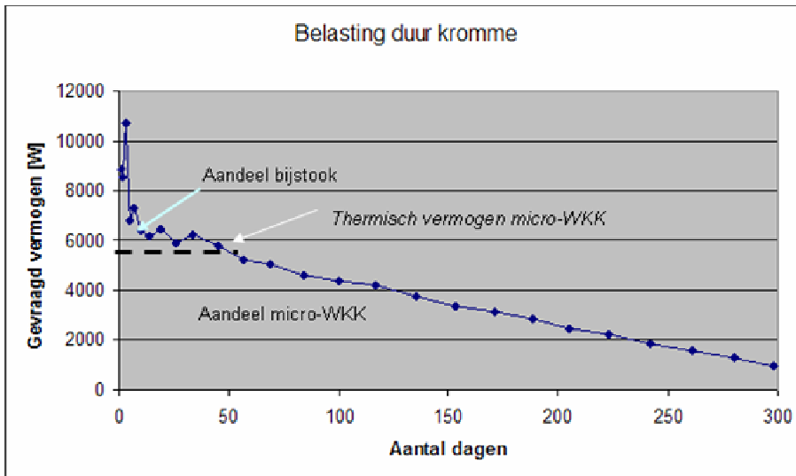
Figuur 3.4: Belasting-duur-kromme voor warmtevraag van 60.000 MJ/jaar
