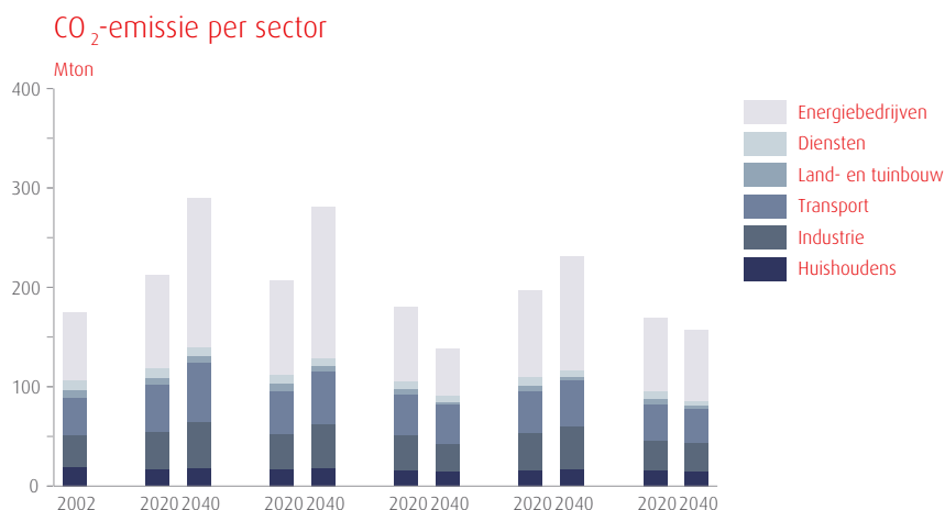
Figuur 6.21 CO 2 -emissie door energiegebruik naar sector.
