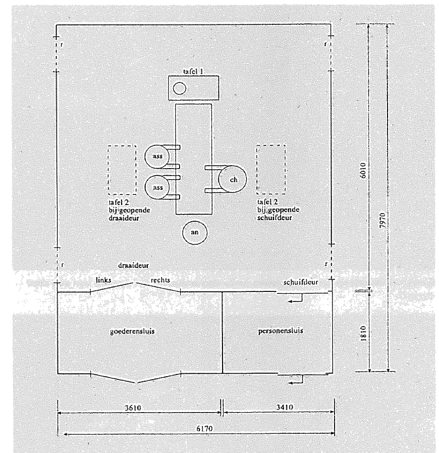
Plattegrond van de cleanroom
