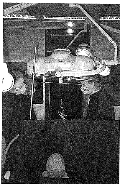
Lamppositie B met één lamp boven de borst en één lamp schuin achter de chirurg -FIGUUR 5-
