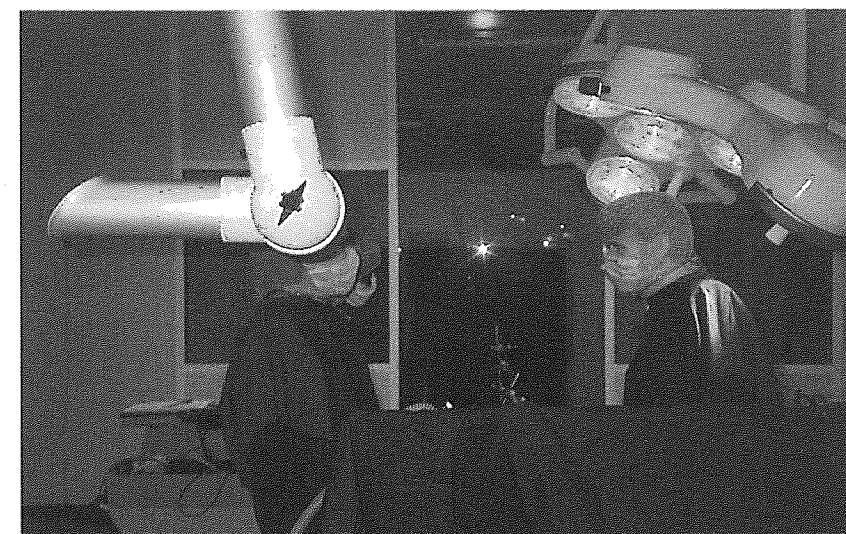
Lamppositie C met lampen schuin achter de chirurg -FIGUUR 6-
