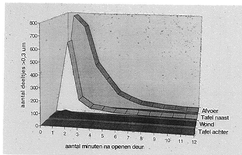
Concentratieverloop op drie plaatsen in de cleanroom na het openen van een deur -FIGUUR 3-
