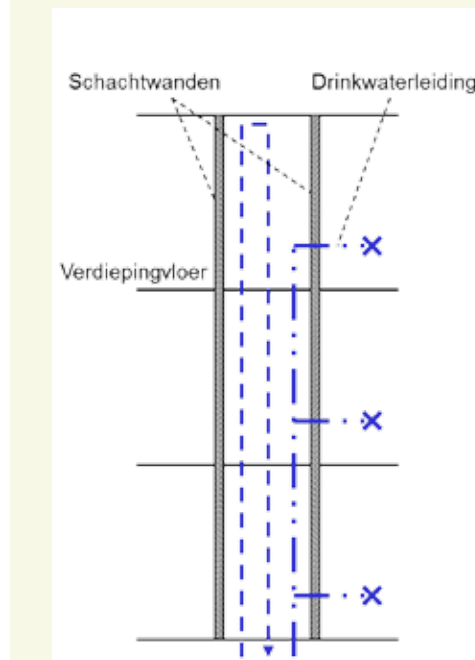
-Figuur 6- Koeling van de schacht met een gekoeldwatersysteem
