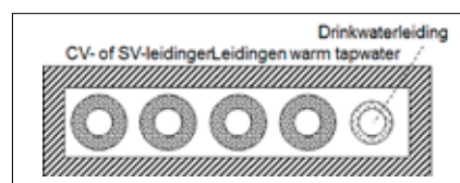
-Figuur 3- Cv- of sv-leidingen en leidingen circulerend warm tapwater in schacht
