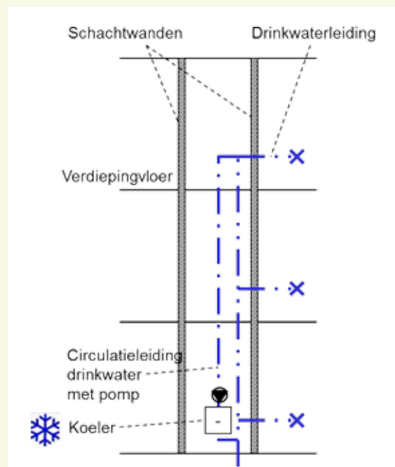
-Figuur 8- Gekoelde circulatieleiding
