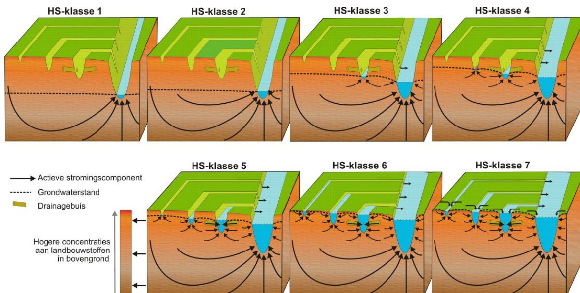
Figuur 4.2: Visualisatie van het conceptuele model voor de relatie tussen grond- en oppervlaktewater; grondwaterstromingscomponenten die onder verschillende afvoersomstandigheden (HS-classes) bijdragen aan het oppervlaktewater
