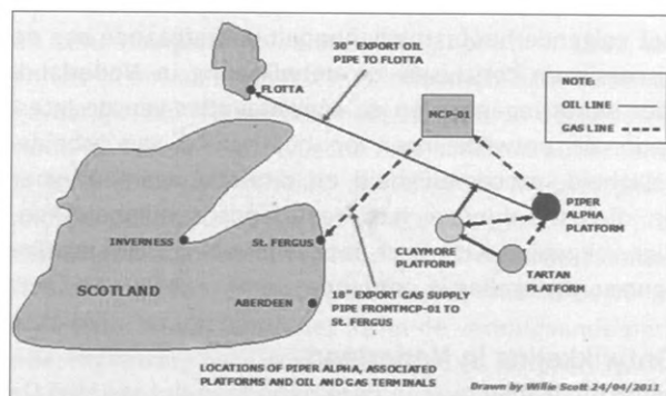
Figuur 11 De verbindingen tussen Occidental platforms
