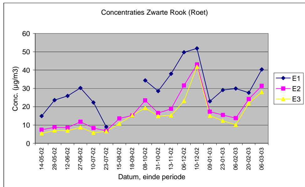
Figuur 6a Resultaten zwarte rook metingen op de meetlocaties E1, E2 en E3: de datum voor de meetpunten in de grafiek geeft de einddatum van de meetperiode aan.
