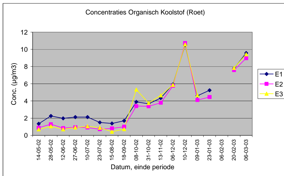
Figuur 6c Resultaten organisch koolstof concentraties ( \mu\text{g koolstof/m}^3 ) op de meetlocaties E1, E2 en E3: de datum voor de meetpunten in de grafiek geeft de einddatum van de meetperiode aan.
