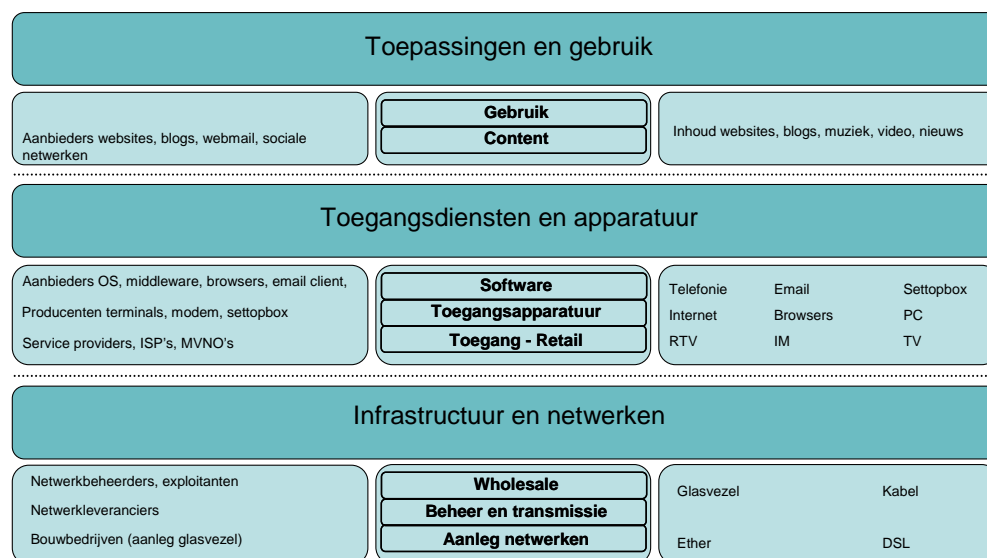
Figuur 1 Lagenmodel
