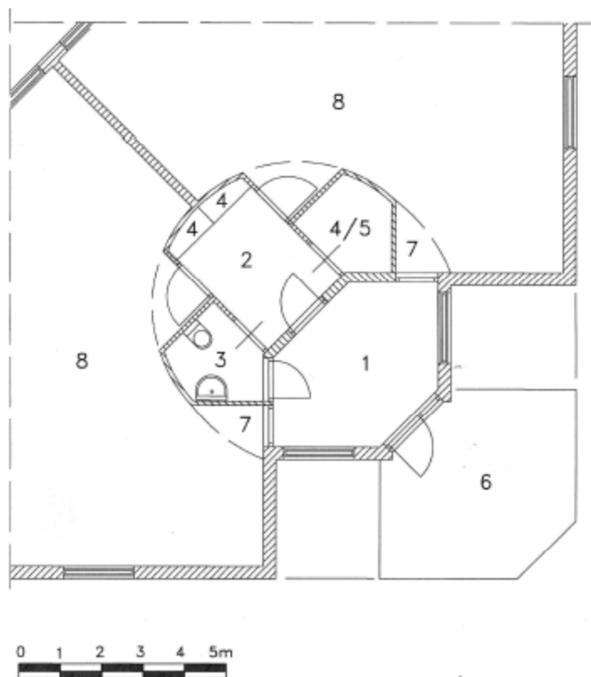
Figuur 3B Voorbeeld van een EBK met toiletruimte.
