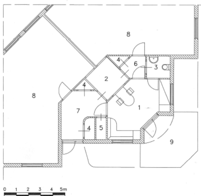
Figuur 3C IC-functie met EBK. De EBK heeft een oppervlakte van circa 18 m 2 en is geleed, waardoor hoeken met een specifieke gebruiksfunctie (rusten, eten, zitten) mogelijk zijn. Ook is een buitenruimte aanwezig die deels overkapt is (zie verder bijlage C).
