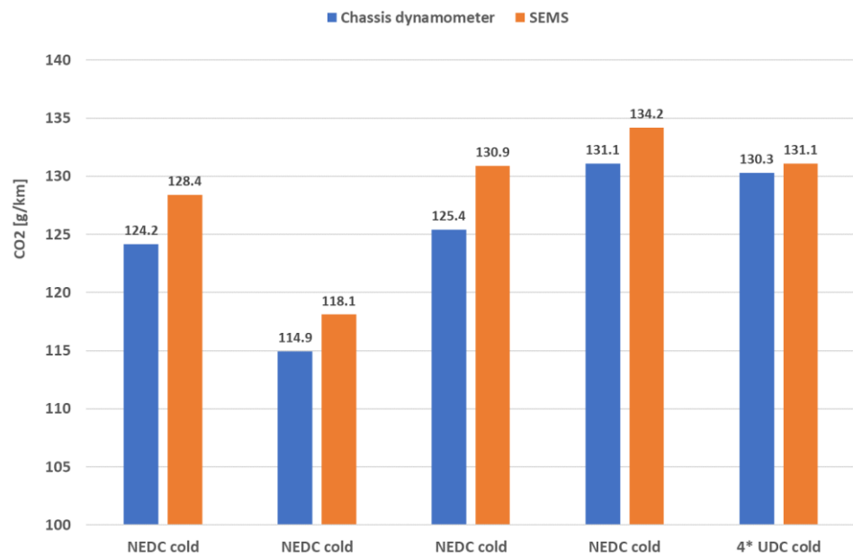
Figuur 4-28: CO 2 emissies met motorkalibratie 1 van verschillende rollenbanktesten gemeten met meetapparatuur van de rollenbank (chassis dynamometer) en met SEMS
