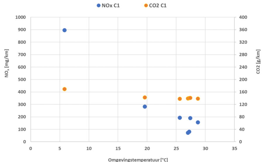
Figuur 4-2: Gecorrigeerde NO x en CO 2 emissies van NEDC testen met koude start gemeten op de testbaan met motorkalibratie 1 bij verschillende omgevingstemperaturen.
