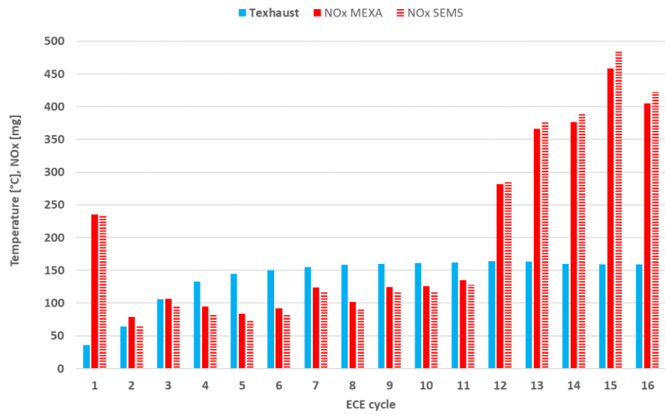
Figuur 5-12: NO x emissies gemeten met rollenbank analysator (MEXA) en met SEMS per ECE cyclus met motorkalibratie 2 van een 4*UDC test met koude start, start-stop actief, uitgevoerd op 11-12-2018. De test is uitgevoerd op de rollenbank met een omgevingstemperatuur van 23 °C. Preconditionering 3*EUUDC met warme start op 10-12-2018 met 3 LNT regeneraties in de tweede en derde EUUDC cyclus.
