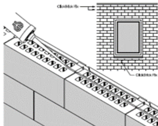
Figuur D.4 Productblad ClickBrick (4/4)
