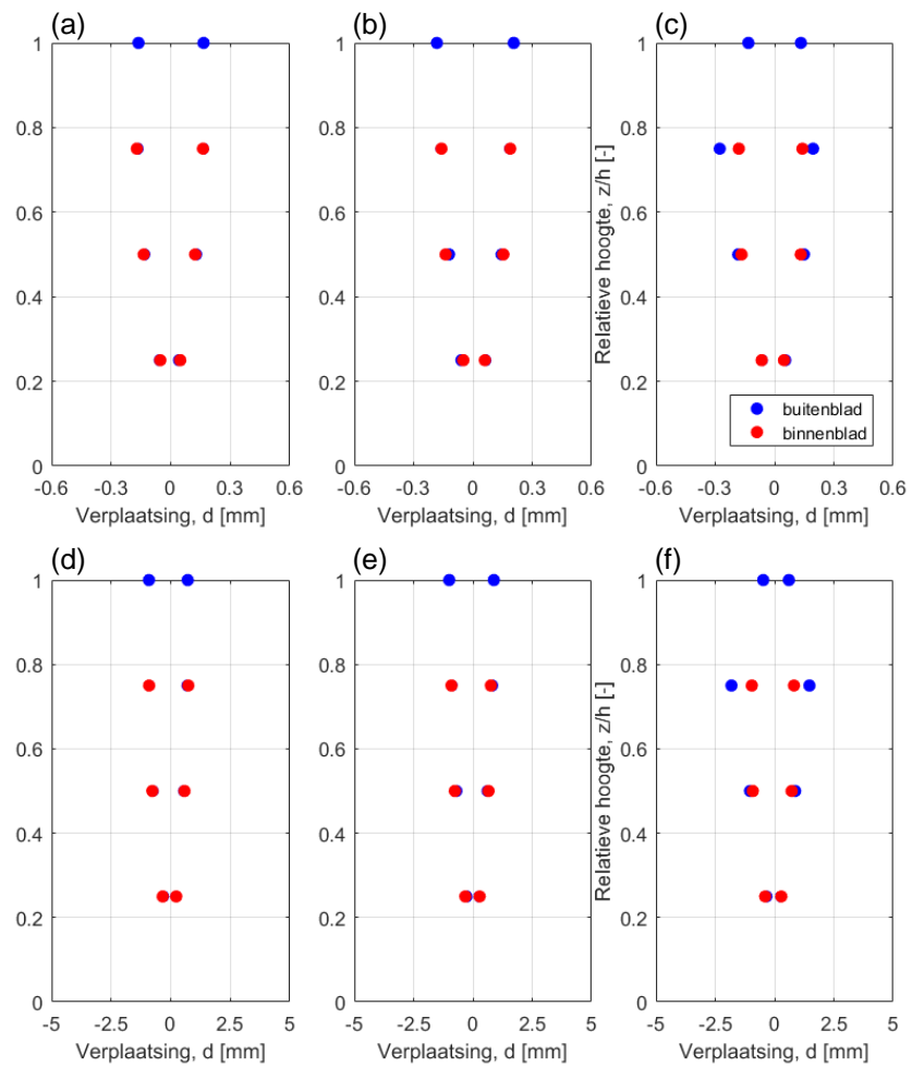
Figuur 22 Verplaatsing van de proefstukken op 4 posities over de hoogte: (a) R1 – Gr-1 (20%), (b) R2 – Gr-1 (20%), (c) ClickBrick – Gr-1 (20%), (d) R1 – Gr-1 (100%), (e) R2 – Gr-1 (100%), en (f) ClickBrick – Gr-1 (100%).
