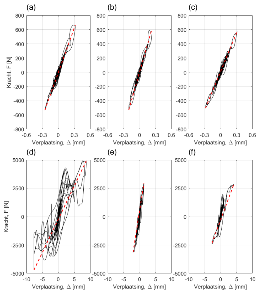
Figuur 29 Grafieken met de kracht op het proefstuk tegen de verplaatsing in het midden van het proefstuk: (a) R1 – Gr-2 (20%), (b) R2 – Gr-2 (20%), (c) ClickBrick – Gr-2 (20%), (d) R1 – Gr-2 (100%), (e) R2 – Gr-2 (100%), en (f) ClickBrick – Gr-2 (100%).
