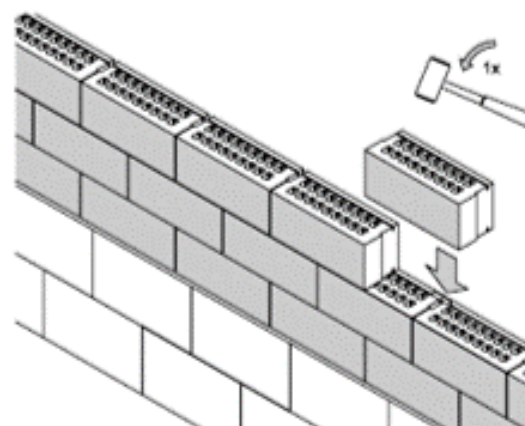
Figuur D.2 Productblad ClickBrick (2/4)
