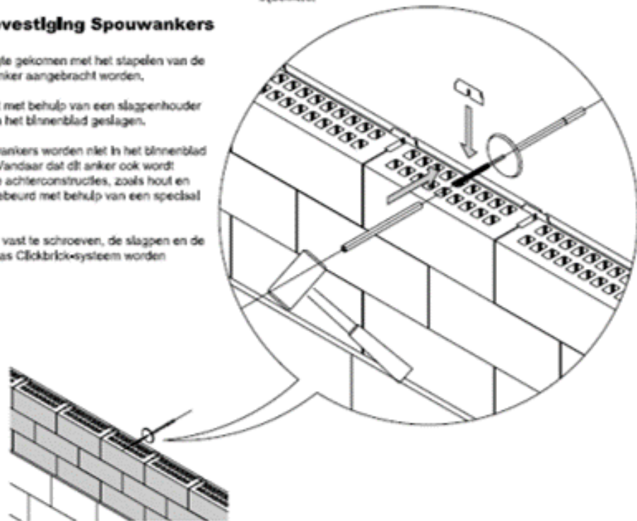
Figuur D.3 Productblad ClickBrick (3/4)
