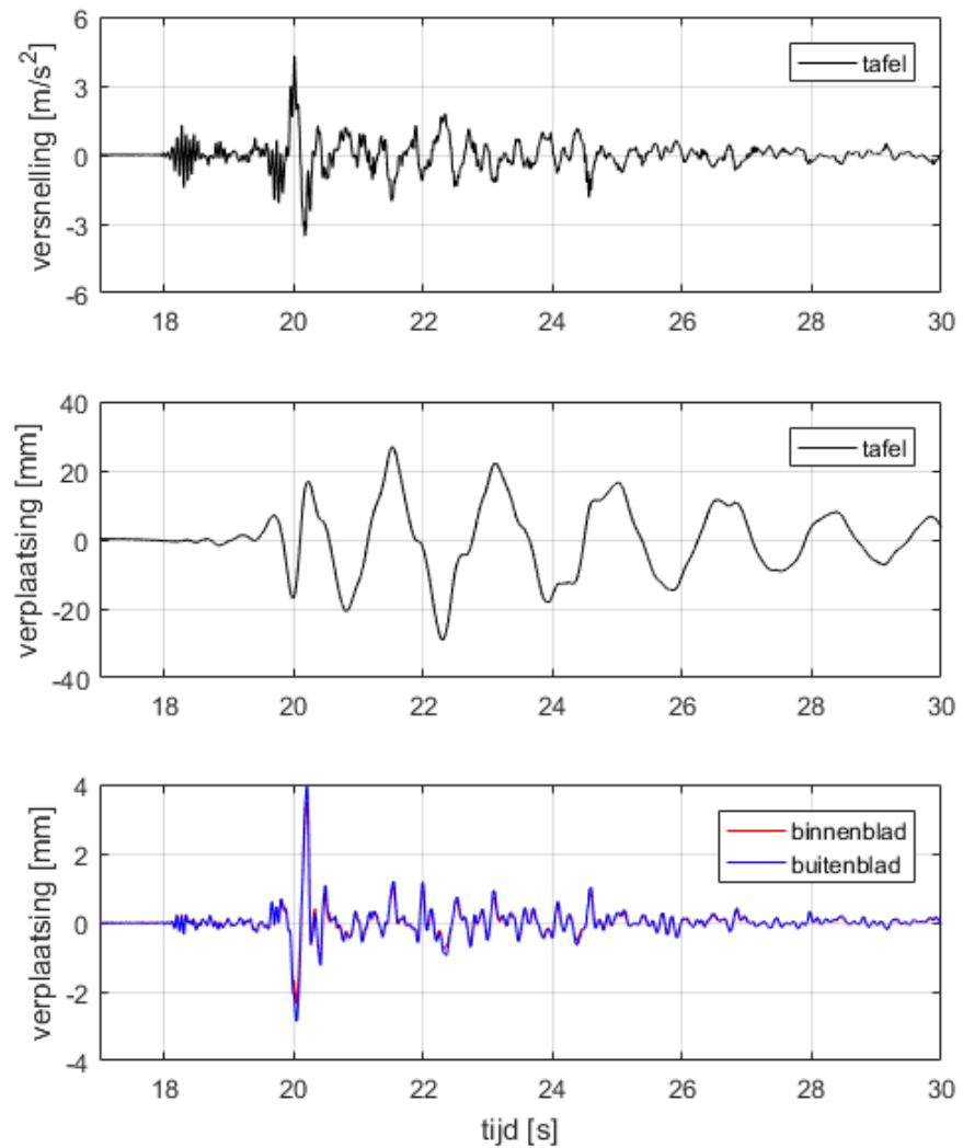
Figuur G.6 Gemeten signalen tijdens een test met Gr-1 (100%) op het ClickBrick proefstuk: (a) het tafel versnellingssignaal, (b) het tafel verplaatsingssignaal, en (c) het relatieve verplaatsingssignaal gemeten in het midden van het binnen- en buitenblad van het proefstuk ten opzichte van de tafel.
