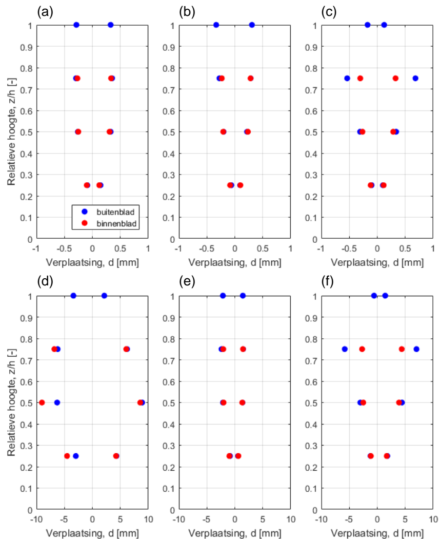
Figuur 28 Verplaatsing van de proefstukken op 4 posities over de hoogte: (a) R1 – Gr-2 (20%), (b) R2 – Gr-2 (20%), (c) ClickBrick – Gr-2 (20%), (d) R1 – Gr-2 (100%), (e) R2 – Gr-2 (100%), en (f) ClickBrick – Gr-2 (100%).
