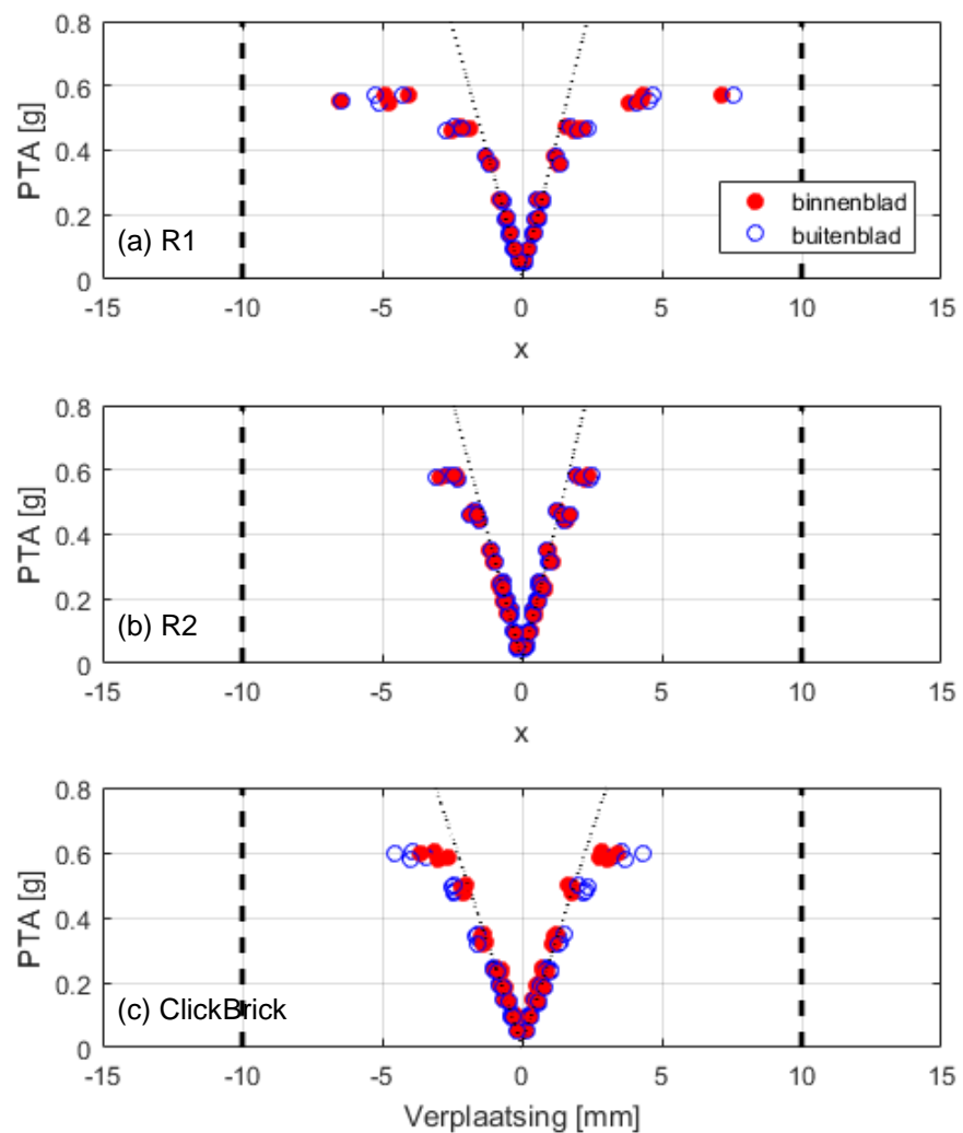
Figuur 20 Verplaatsing midden proefstuk tegen piek tafel versnelling (PTA = Peak Table Acceleration) gemeten met signaal Gr-1: (a) R1, (b) R2, (c) ClickBrick. De zwarte gebroken lijn specificeert het meetbereik van de verplaatsingsopnemers; de zwarte stippellijn is een gefitte lijn op de data met PTA \leq 0.2 g.
