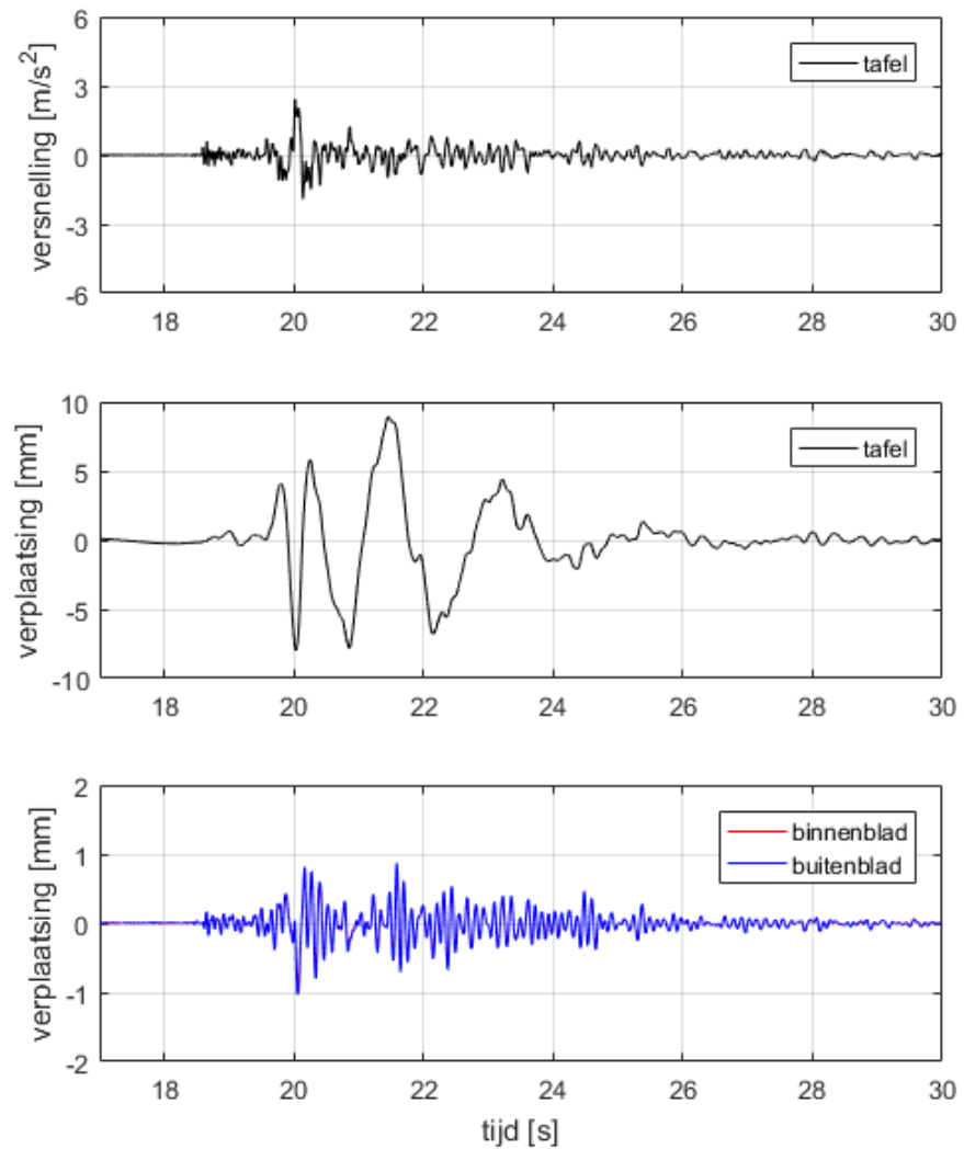
Figuur G.3 Gemeten signalen tijdens een test met Gr-1 (100%) op het ClickBrick proefstuk: (a) het tafel versnellingssignaal, (b) het tafel verplaatsingssignaal, en (c) het relatieve verplaatsingssignaal gemeten in het midden van het binnen- en buitenblad van het proefstuk ten opzichte van de tafel.
