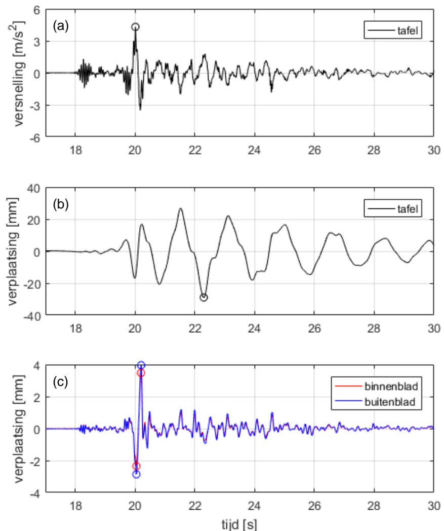
Figuur 25 Gemeten signalen op het ClickBrick proefstuk voor een test met Gr-2 (100%): (a) het tafel versnellingssignaal, (b) het tafel verplaatsingssignaal, en (c) het relatieve verplaatsingssignaal gemeten in het midden van het binnen- en buitenblad van het proefstuk ten opzichte van de tafel.
