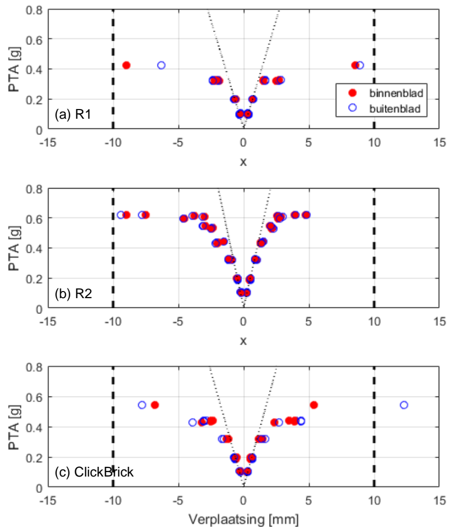
Figuur 26 Verplaatsing midden proefstuk tegen piek tafel versnelling (PTA) gemeten met signaal Gr-2: (a) proefstuk R1, (b) proefstuk R2 en (c) ClickBrick. De zwarte gebroken lijn specificeert het meetbereik van de verplaatsingsopnemers; de zwarte stippellijn is een gefitte lijn op de data met PTA \leq 0.2 g.
