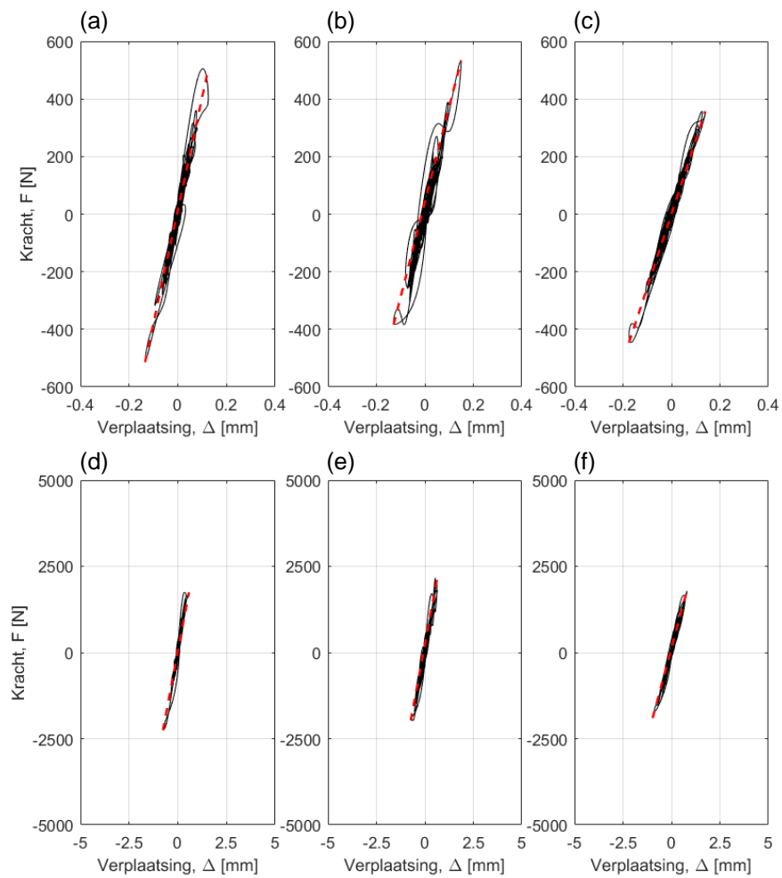
Figuur 23 Grafieken met de kracht op het proefstuk tegen de verplaatsing in het midden van het proefstuk: (a) R1 – Gr-1 (20%), (b) R2 – Gr-1 (20%), (c) ClickBrick – Gr-1 (20%), (d) R1 – Gr-1 (100%), (e) R2 – Gr-1 (100%), en (f) ClickBrick – Gr-1 (100%).
