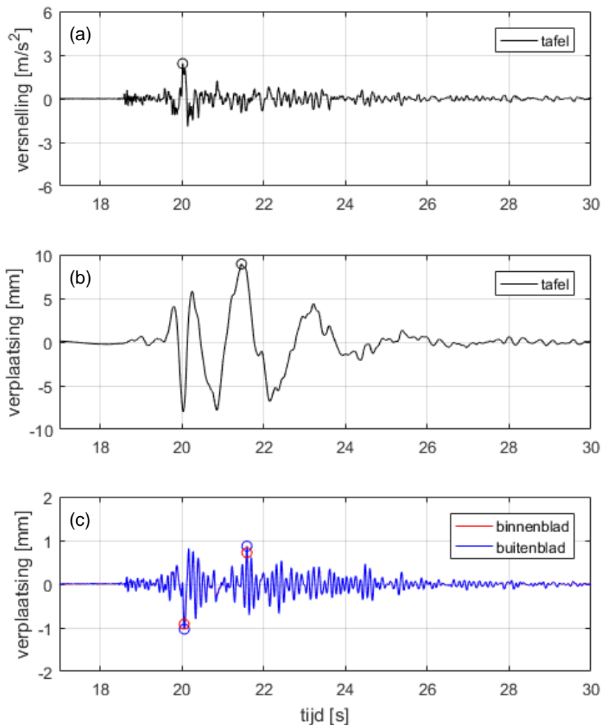
Figuur 19 Gemeten signalen tijdens een test met Gr-1 (100%) op het ClickBrick proefstuk: (a) het tafel versnellings signaal, (b) het tafel verplaatsingssignaal, en (c) het relatieve verplaatsingssignaal gemeten in het midden van het binnen- en buitenblad van het proefstuk ten opzichte van de tafel.
