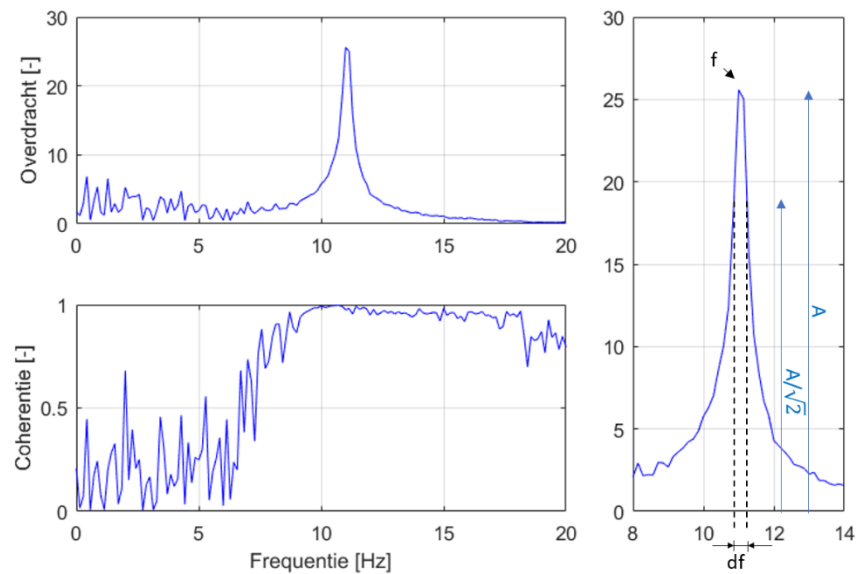
Figuur F.8 Spectra bepaald uit meetdata: (a) overdrachtsspectrum, (b) coherentiespectrum, (c) detail van piek in overdrachtsspectrum.
