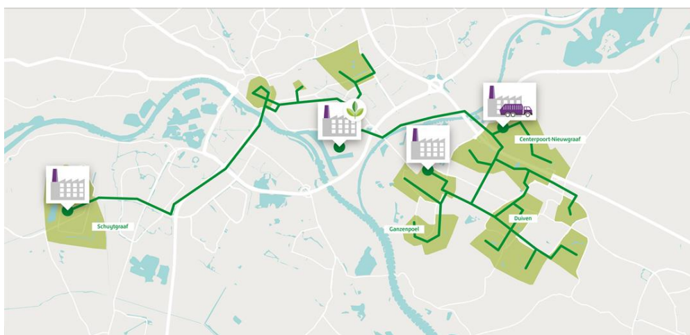
Figuur 3.13 Warmtenet Arnhem, Duiven en Westervoort (Nuon, 2017). Het groen gearceerde deel geeft het leveringsgebied van Nuon weer
