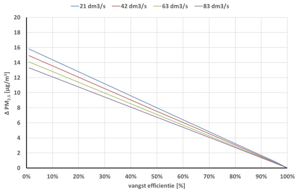
Figuur 4 gemiddelde PM 2,5 verhoging over de verblijfsduur in de woning bij een PM 2,5 emissie van 25 mg als functie van vangstefficiëntie en afzuigdebiet tijdens koken. Hier is nog geen relatie gelegd tussen vangstefficiëntie en afzuigdebiet van een afzuigkap.
