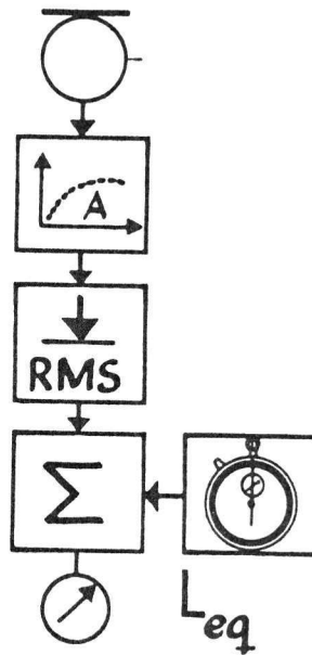
Figuur 19: Schema geluidexpositiemeter.
