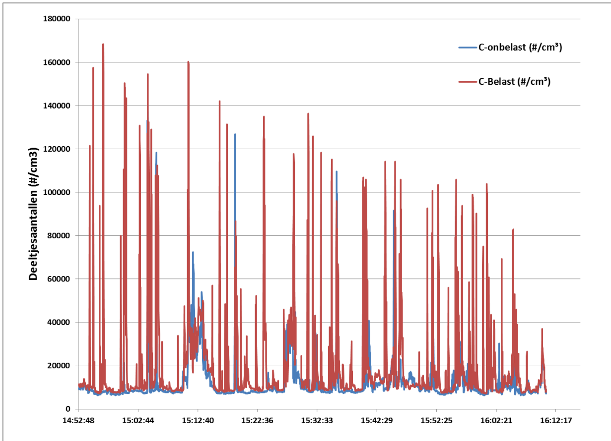
Figuur 24: Trend van de deeltjes aantallen boven en benedenwinds van het fietspad op de Vleutenseweg Onbelast is bovenwinds.
