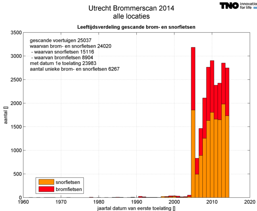
Figuur 16: De verhouding tussen snor- en bromfietsen over de diverse jaren van eerste toelating.
