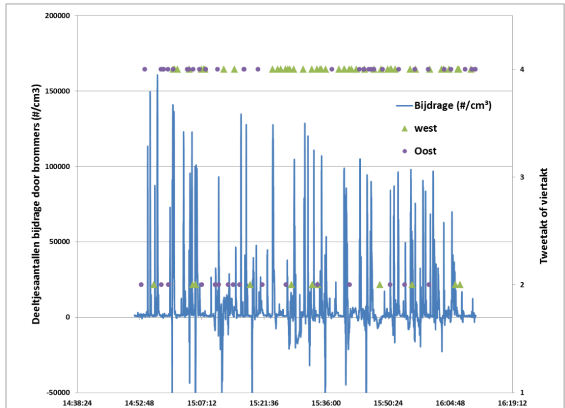
Figuur 25: Bijdrage van brommers aan de deeltjesaantallen benedenwinds van het fietspad. De groene driehoekjes zijn geregistreeerde brommers die rijden in de westelijke richting. De paarse rondjes zijn brommers in de oostelijke richting. Bij de brommers is op de rechter-as onderscheid gemaakt tussen twee- en viertakt.
