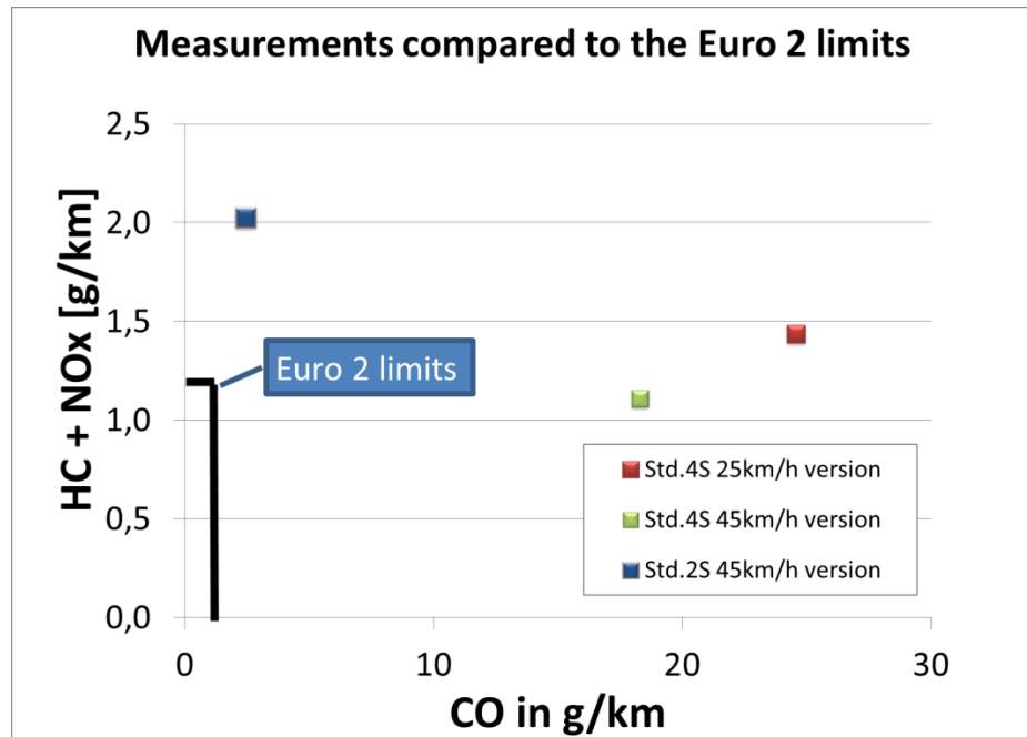
Figuur 7: Emissies van zowel de twee- als viertaktbrommer in originele conditie. De viertaktbrommer is zowel als snorfiets als brommer variant gemeten.
