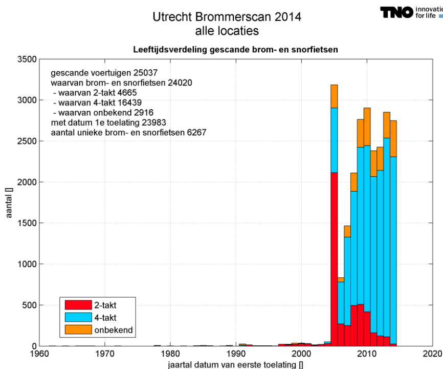
Figuur 5: De verhouding van tweetakt- en viertaktbrommers in Utrecht, uitgesplitst naar datum eerste toelating. De meeste brommers van bouwjaar 2005 en eerder zijn opgenomen onder 2005.
