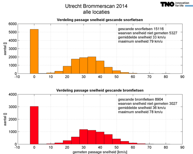
Figuur 6: Snelheidsverdeling van snor- en bromfietsen. Snelheid 0 betekent dat de betreffende meting niet betrouwbaar of niet gelukt is.
