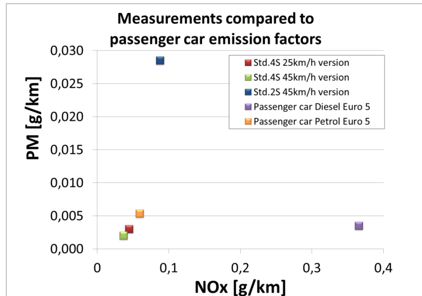
Figuur 8: Fijnstof en NO x emissies van de gemeten brommers en fijnstof en NO x emissiefactoren van personenwagens
