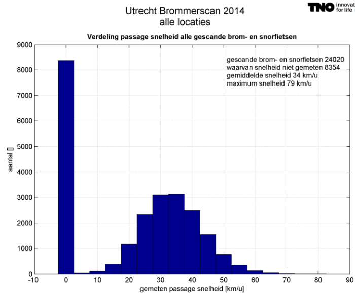
Figuur 21: Snelheidsverdeling van de brom- en snorfietsen.
