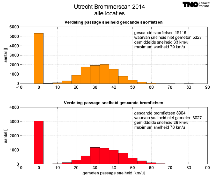
Figuur 22: Snelheidsverdeling van snor- en bromfietsen
