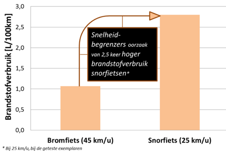
Figuur 10: Sommige typen snelheidsbegrenzer zorgen voor een wel 2,5 maal zo hoog brandstofverbruik van snorfietsen.
