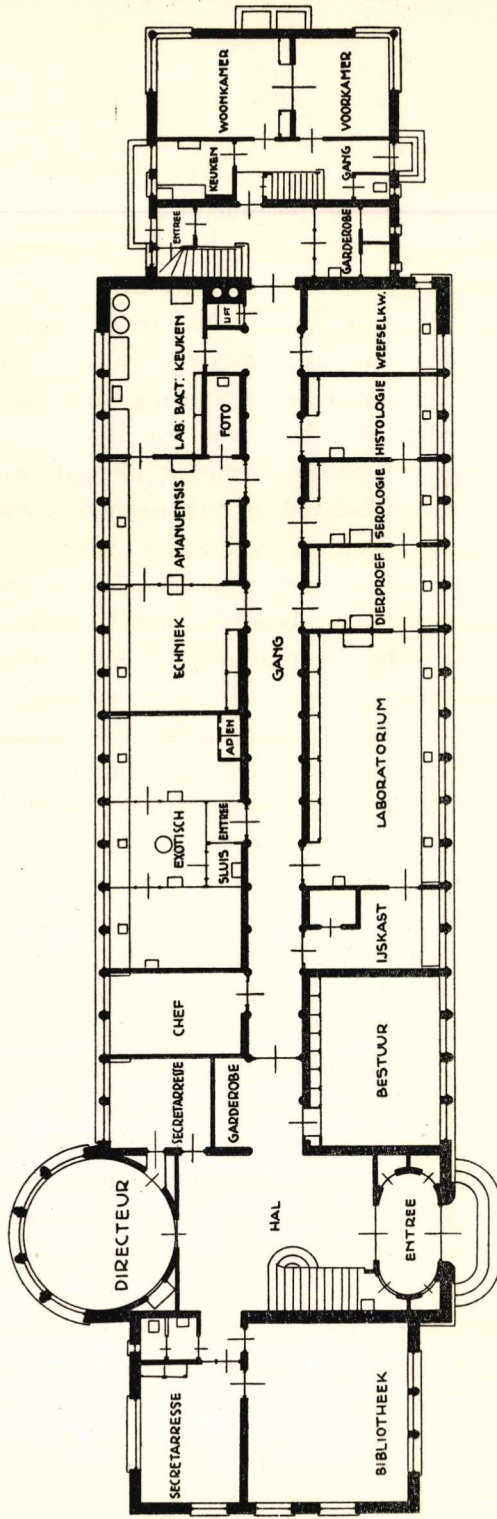
Fig. 2. Hoofdgebouw, begane grond.
